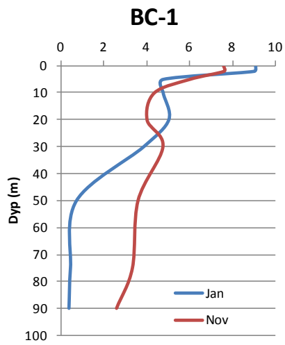
Figur 28. Oksygenprofil fra stasjon BC-1 i Frierfjorden 2013. I figuren er vist resultater fra januar og november.
