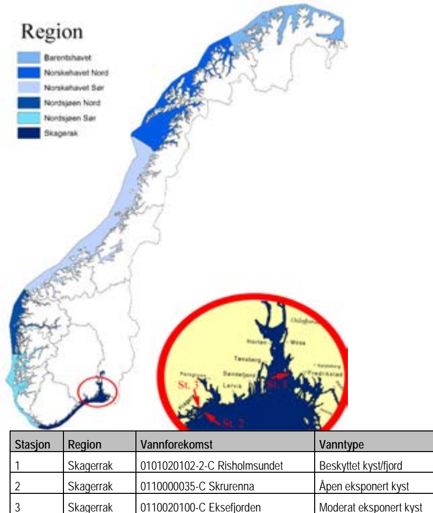
Figur 1. Oversikt over regionene i Norge i hht. vannforskriften hvor undersøkelsesområdene er markert med rød sirkel (kart hentet fra vannportalen.no). Og en oversikt over hvilken vannforekomst de tre nedre voksegrense-stasjonene undersøkt i 2013 ligger i og hvilken vanntype de tilhører (fra vann-nett.no).
