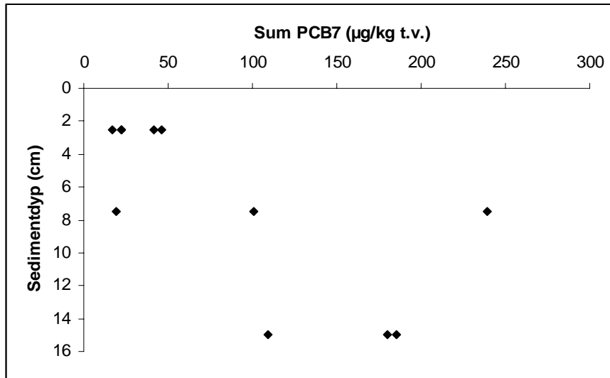
Figur 6. Konsentrasjonen av \Sigma PCB_7 (summen av 7 enkeltforbindelser av PCB) i 3 ulike dybdeavsnitt (1- 5 cm, 5-10 cm og 10-20 cm) i sediment fra Bekkelagsbassenget. På y-aksen er midlere dyp for hvert av dybdeavsnittene avmerket.
