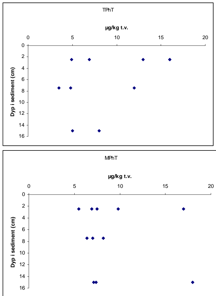
Figur 13. Konsentrasjonen ( \mu\text{g}/\text{kg t.v.} ) av TPhT=trifenyltinn og MPhT=monofenyltinn. i 3 ulike dybdeavsnitt (1- 5 cm, 5-10 cm og 10-20 cm) i sediment fra Bekkelagsbassenget. På y-aksen er midlere dyp for hvert av dybdeavsnittene avmerket.
