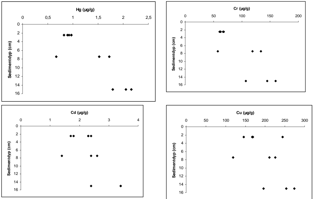
Figur 4. Konsentrasjonen ( \mu\text{g/g} t.v.) av kvikksølv (Hg), krom (Cr), kadmium (Cd) og kobber (Cu) i 3 ulike dybdeavsnitt (1-5 cm, 5-10 cm og 10-20 cm) i sediment fra Bekkelagsbassenget. På y-aksen er midlere dyp for hvert av dybdeavsnittene avmerket.
