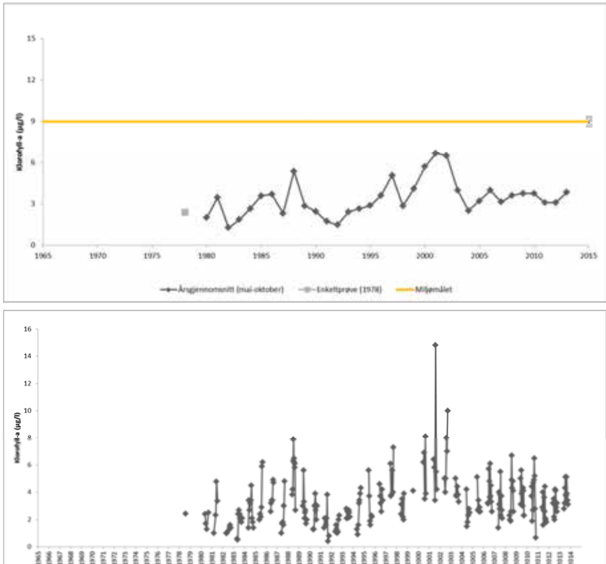
Figur 14. Øverst: Utvikling av klorofyll-a konsentrasjonen i overflatelaget i Femsjøen fra 1978 til 2013. Årgjennomsnitt er fra perioden mai til oktober. Fra 1970-tallet er det noen år der det kun er en prøve i perioden mai-oktober. Miljømålet for klorofyll-a er på 9 µg/l for vanntype L-N3. Nederst: Enkeltverdier for klorofyll-a fra hvert år.
