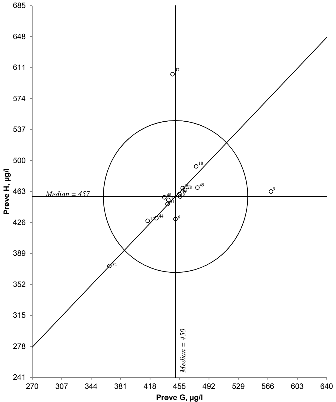
Figur 41. Youndendiagram for totalnitrogen, prøvepar GH Akseptansesgrensen, angitt med en sirkel, er 20 %
