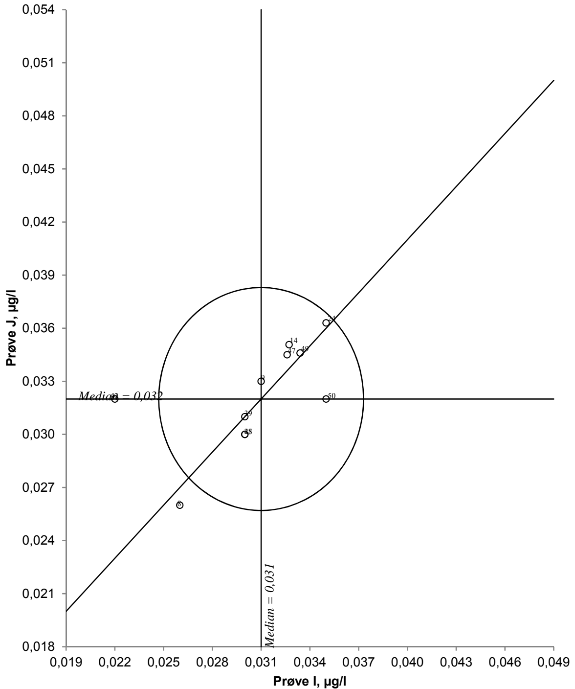
Figur 48. Youndendiagram for kadmium, prøvepar IJ Akseptansgrensen, angitt med en sirkel, er 20 %
