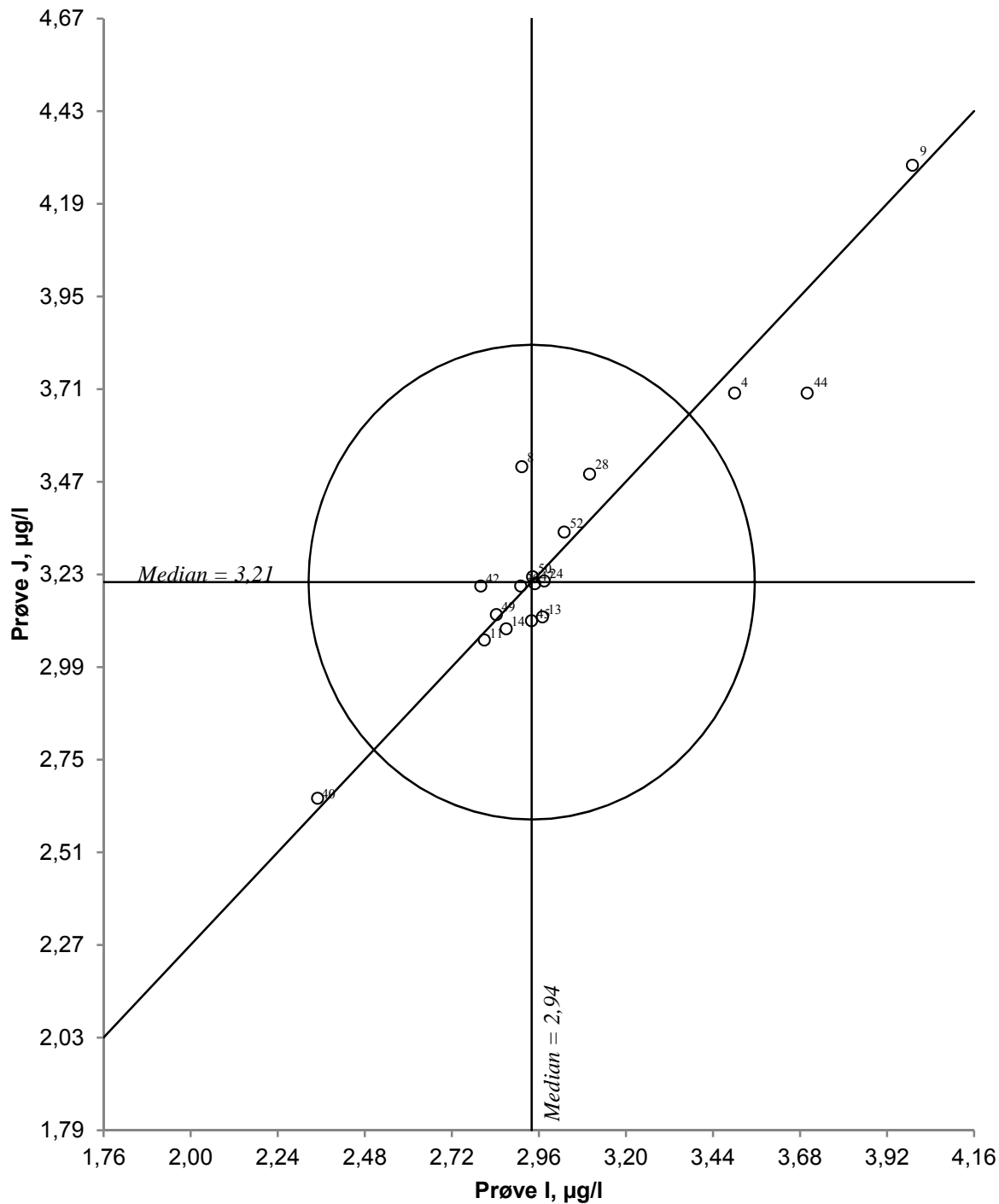
Figur 44. Youtendigram for bly, prøvepar IJ Akseptansgrensen, angitt med en sirkel, er 20 %
