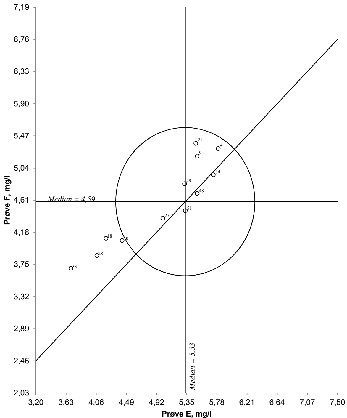
Figur 28. Youndendiagram for kjemisk oksygenforbruk, COD/Mn, prøvepar EF Akseptansesegrensen, angitt med en sirkel, er 20 %
