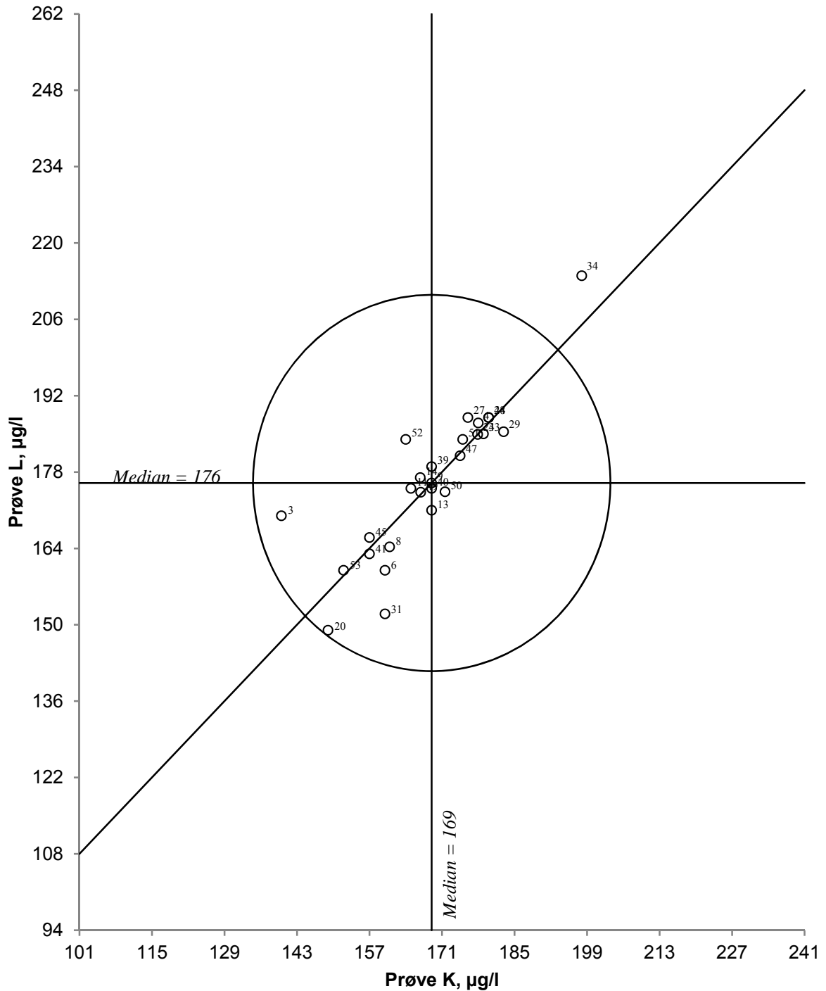
Figur 47. Youndendiagram for jern, prøvepar KL Akseptansesgrensen, angitt med en sirkel, er 20 %
