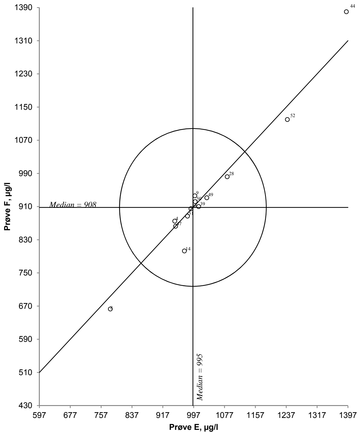
Figur 40. Youtenddiagram for totalnitrogen, prøvepar EF Akseptansgrensen, angitt med en sirkel, er 20 %
