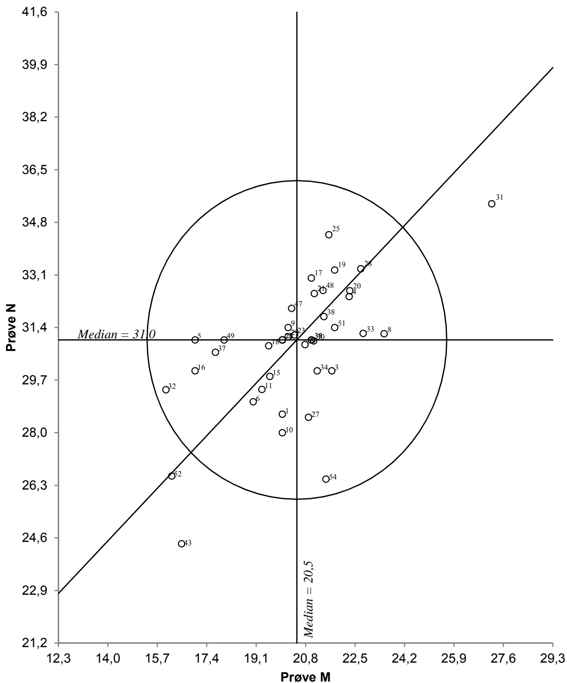
Figur 6. Youtenddiagram for fargetall, prøvepar MN Akseptansesgrensen, angitt med en sirkel, er 20 %
