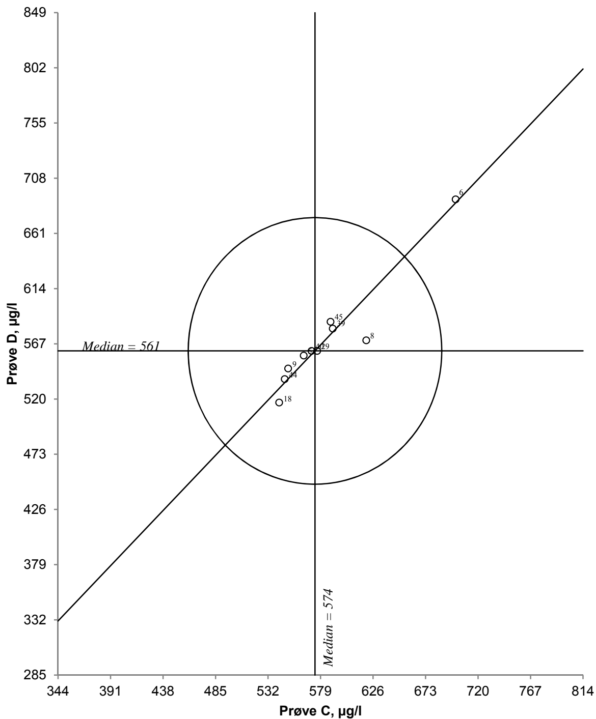
Figur 37. Youndendiagram for nitrat, prøvepar CD Akseptansgrensen, angitt med en sirkel, er 20 %
