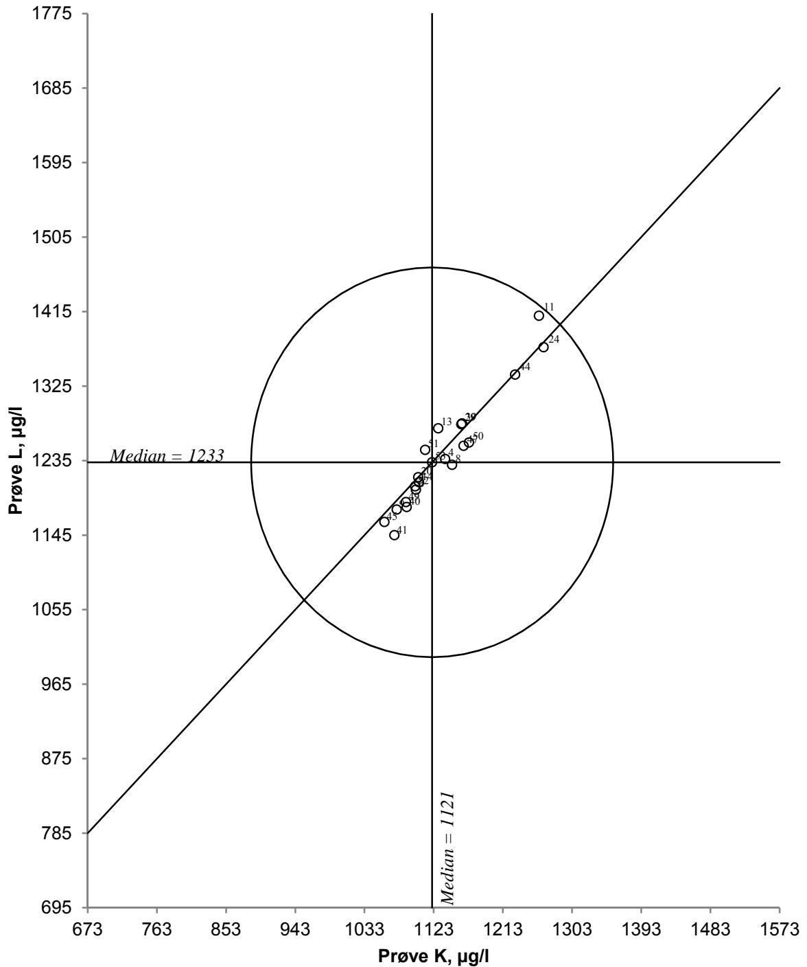
Figur 51. Youndendiagram for kobber, prøvepar KL Akseptansgrensen, angitt med en sirkel, er 20 %
