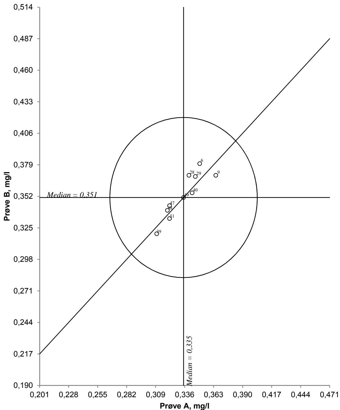
Figur 24. Youdendiagram for fluorid, prøvepar AB Akseptansesgrensen, angitt med en sirkel, er 20 %
