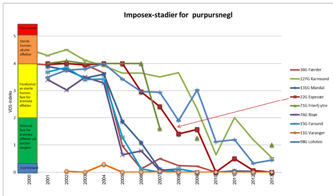
Figur 14. Utvikling av VDS indeksverdi (Vas Deference Sequence Index) for imposex i purpursnegl på 9 lokaliteter langs norskekysten i perioden 1991 – 2013 (Green et al. 2014). Stasjonen mest sammenliknbar med Fedje, Espevær, er indikert med pil.
