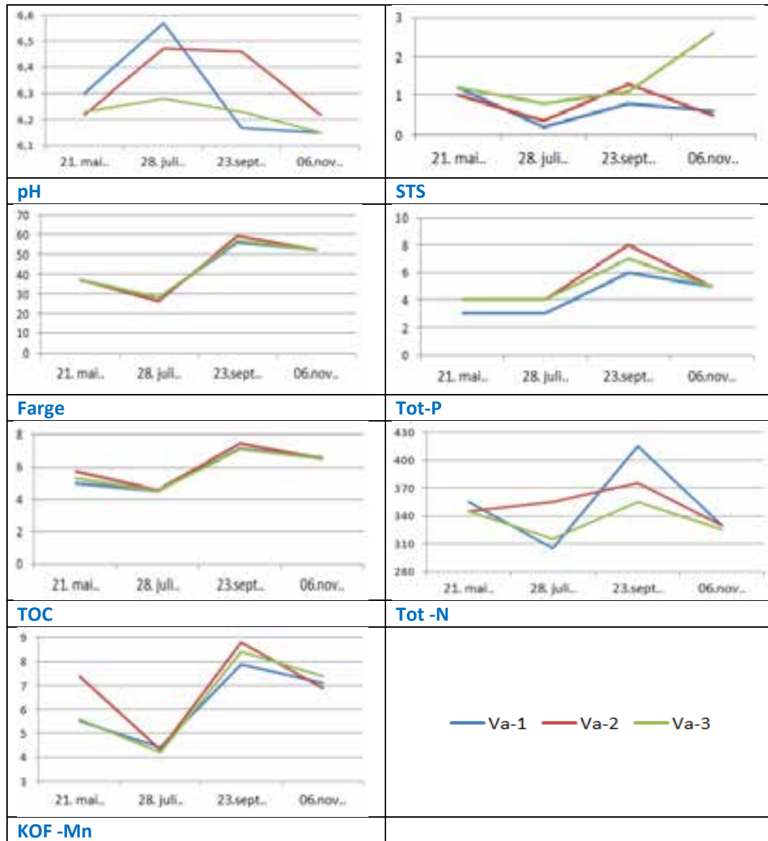
Figur A1. Resultater fra overvåkingen av Vadfoss- og Kammerfosselven ved Vafos Pulp AS i 2015. Kurvene viser utviklingen nedover i vassdraget fra stasjon Va-1 oppstrøms til St. Va-2 og Va-3 nedstrøms bedriften, ved hver prøvetaking.
