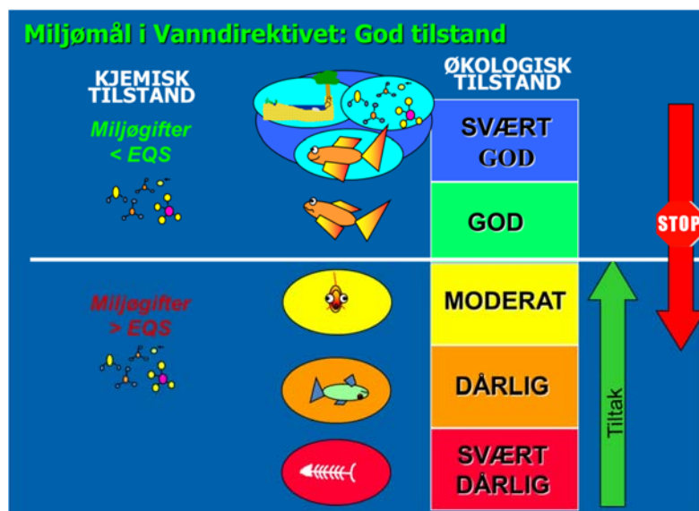
Figur 1. Prinsippeskisse for klassifisering av økologisk og kjemisk tilstand. Se tekst for nærmere forklaring.
