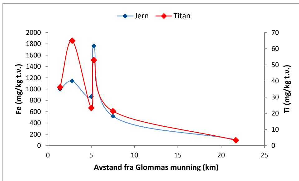
Figur 10. Konsentrasjonen av jern (Fe) og titan (Ti) i blæretang i ulike avstand fra Kaldera (fyrlykt på Kråkerøy Østerevna) i 2015.
