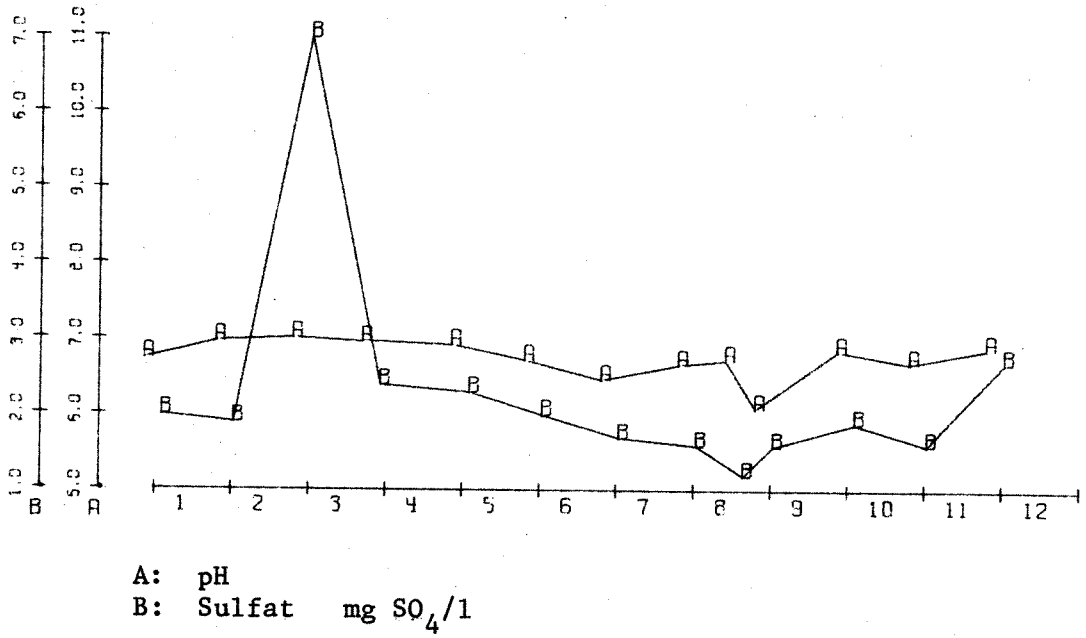
Fig. 28. Stasjon El. Grafisk fremstilling av analyseresultater 1977. pH og sulfat.
