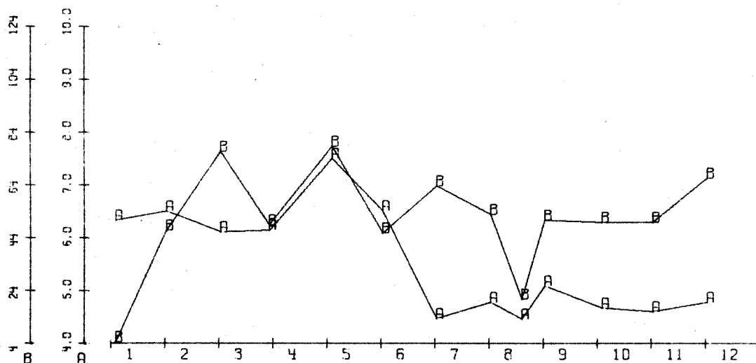
Fig. 22. Stasjon B5. Grafisk fremstilling av analyseresultater 1977. pH og sulfat.
