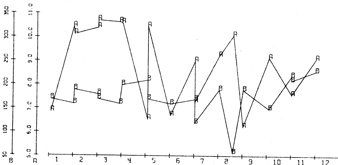
Fig. 19. Stasjon B3. Grafisk fremstilling av analyseresultater 1977: pH og sulfat.
