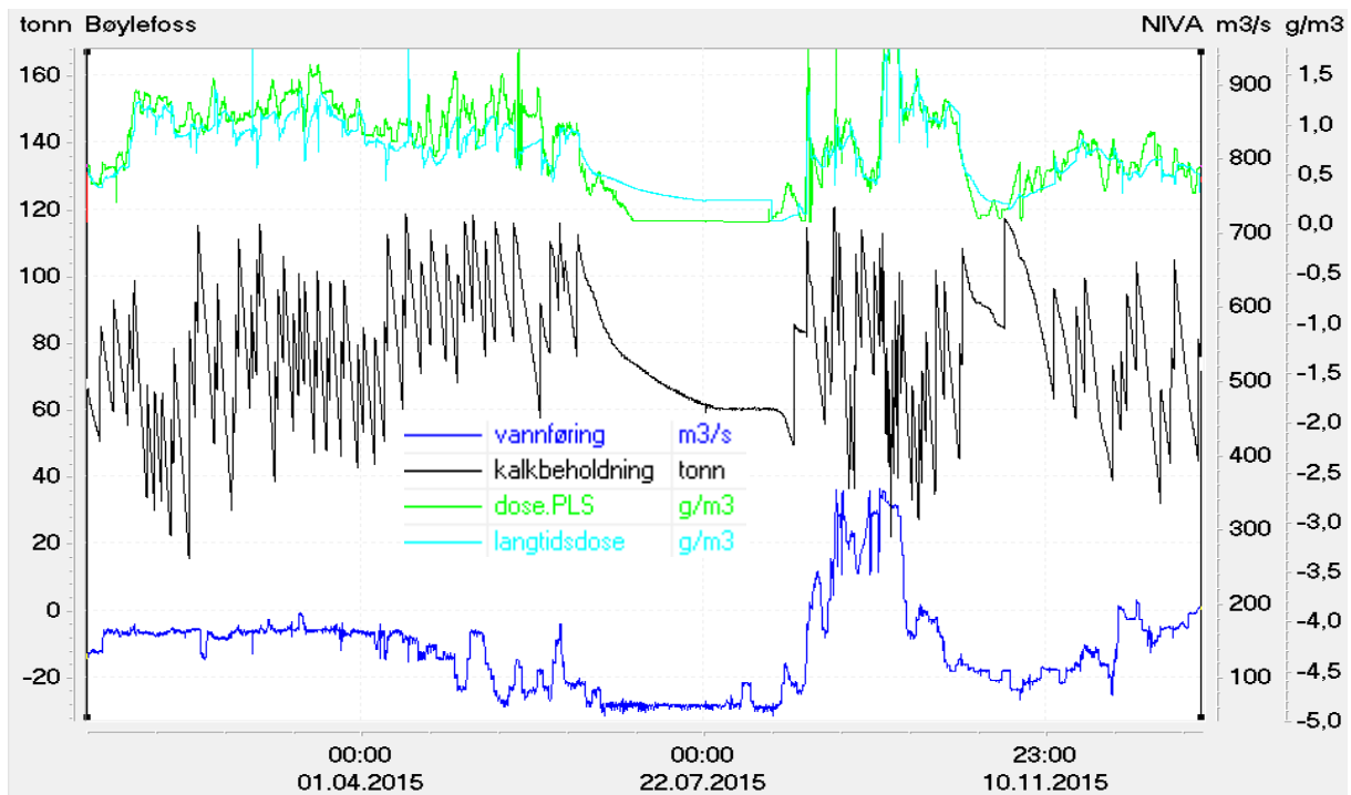
Figur 4. Vannføring, kalkbeholdning, kalkdoser som PLS-dose (styringsdose) og langtidsdose ved Bøylefoss doseringsanlegg i 2105. Figuren viser en høy dosering vår og høst, samt at det doseres kalk selv om styringssignalet indikerer ingen kalkdosering første del av sommeren.
