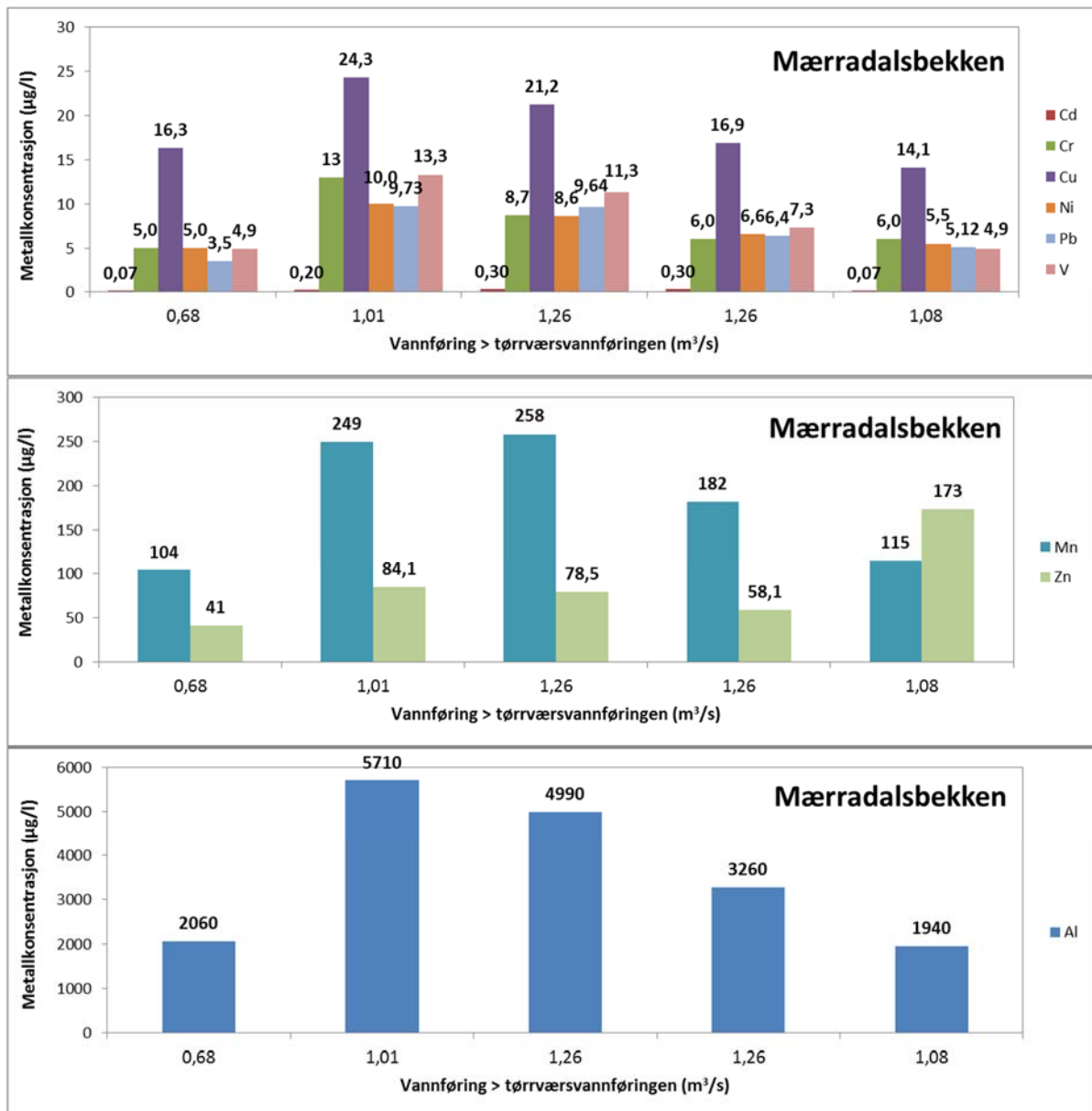
Figur 3. Metallkonsentrasjoner (partikkelbundet og løst) og vannføring over tørrværsvannføringen i Mærradalsbekken i løpet av prøvetakingsperioden.
