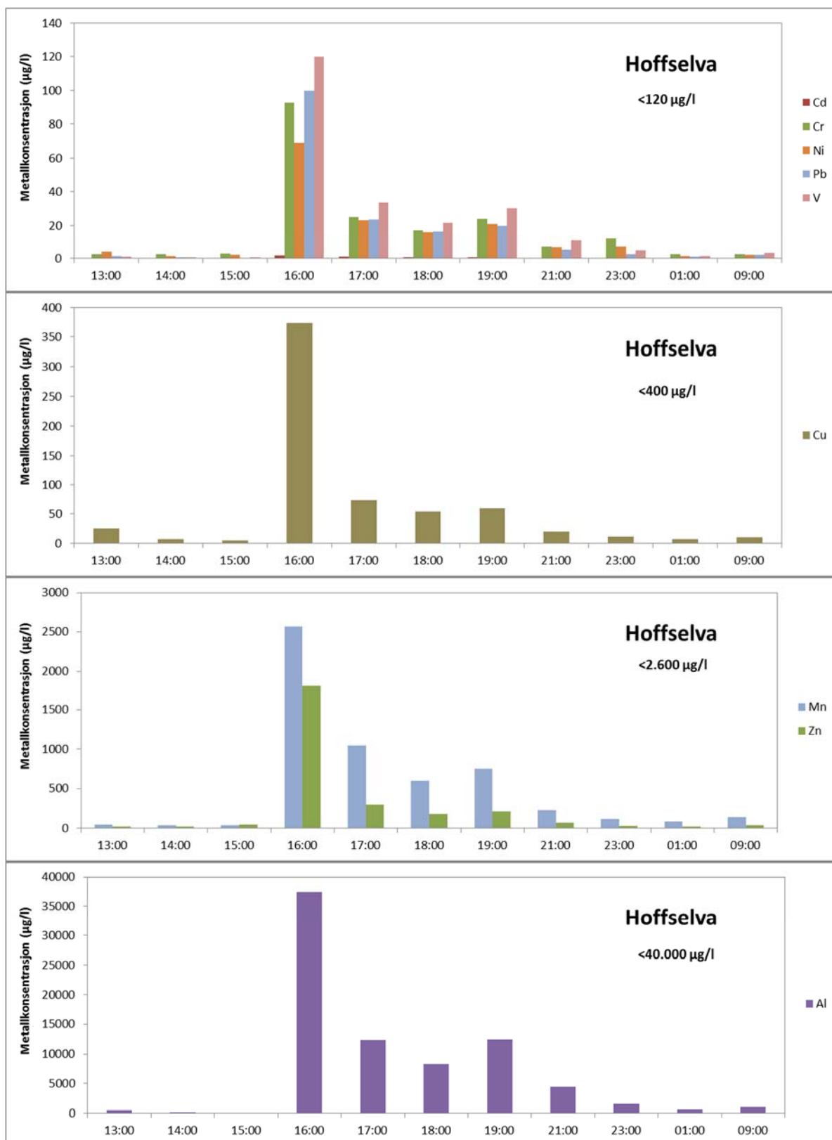
Figur 3. Metallkonsentrasjoner i Hoffselva i løpet av prøvetakingsperioden.
