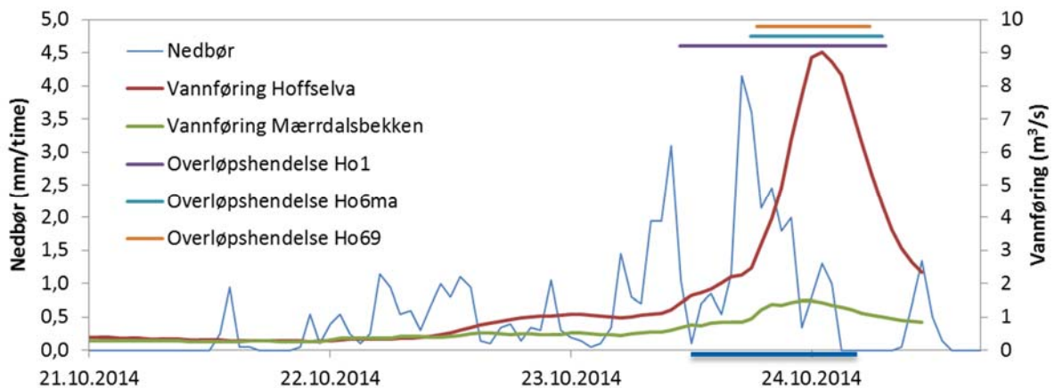
Figur 2. Nedbørshendelsen 21-24.10 2014. Nedbør i perioden, målt vannføring i Hoffselva og Mærradalsbekken og registrerte overløpshendelser (sammenhengende mer enn 20 min). Prøvetaksperioden (fra 23.10 kl. 15 til 24.10 kl 04) er markert med blå vannrett strek.
