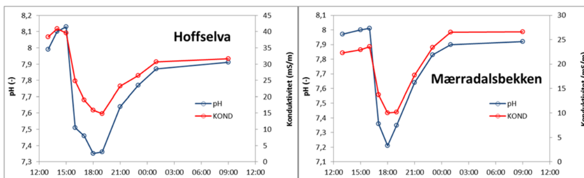
Figur 13. Resultater fra analyse pH og konduktivitet i timesblandprøvene tatt ut under prøvetaksingsperioden i Hoffselva og i Mærradalsbekken.
