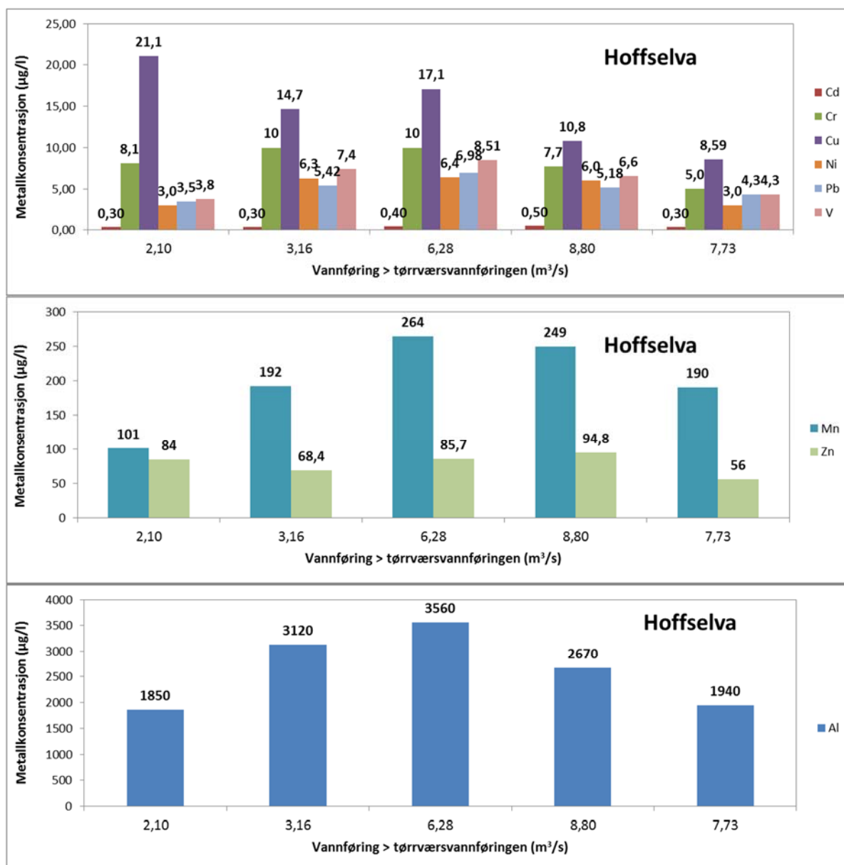
Figur 4. Metallkonsentrasjoner (partikkelbundet og løst) og vannføring over tørrværsvannføringen i Hoffselva i løpet av prøvetaksperioden.
