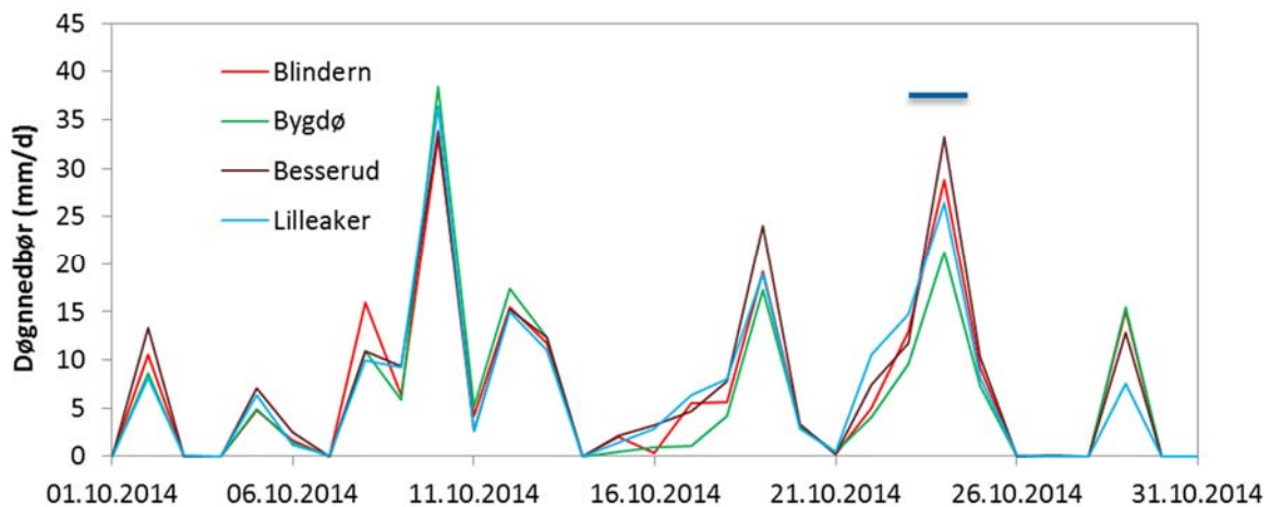
Figur 1. Registrert nedbør ved 4 målestasjoner i rimelig nærhet til Hoffselva og Mærradalsbekken i oktpber 2014. Prøvetaksperioden (fra 23.10 kl. 15 til 24.10 kl 04) er markert med blå vannrett strek.
