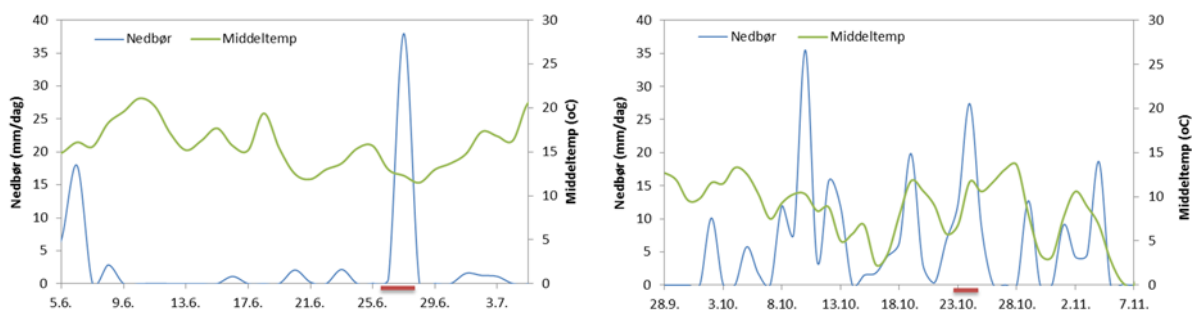
Figur E1. Nedbøren i juni 2014 (venstre) og i oktober 2014 ut fra gjennomsnittet for observasjoner gjort ved værstationene 18700 Blindern, 18815 Bygdø, 18920 Besserud og 18980 Lilleaker. Døgntemperatur er gitt for Oslo-Blindern.
