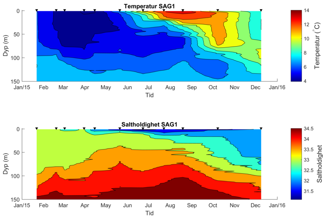
Figur 10. Temperatur (°C) og saltholdighet i 2015 ved stasjon SAG1 i Sagfjorden. Pilsymbolene (▼) på grafenes topplinje angir tidspunkt for de utførte målingene gjennom året.
