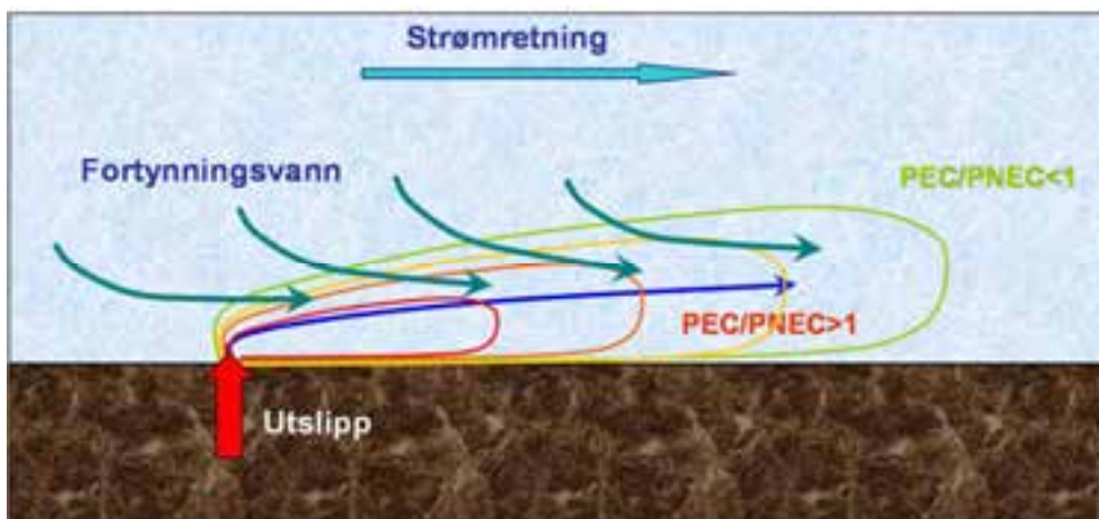
Figur 2. Skjematisk skisse av blandingsforløp og influensområde av et utslipp til sjø. Utslippet følger strømmen og blandes gradvis med omgivende vann. Stoffet i utslippet fortynnes, og konsentrasjonen ( PEC ) vil etter hvert nærme seg grenseverdi for effekter ( PNEC ). Når PEC < PNEC er det ikke lenger risiko for toksiske virkninger. Grønn linje angir derfor grensen for influensområdet.
