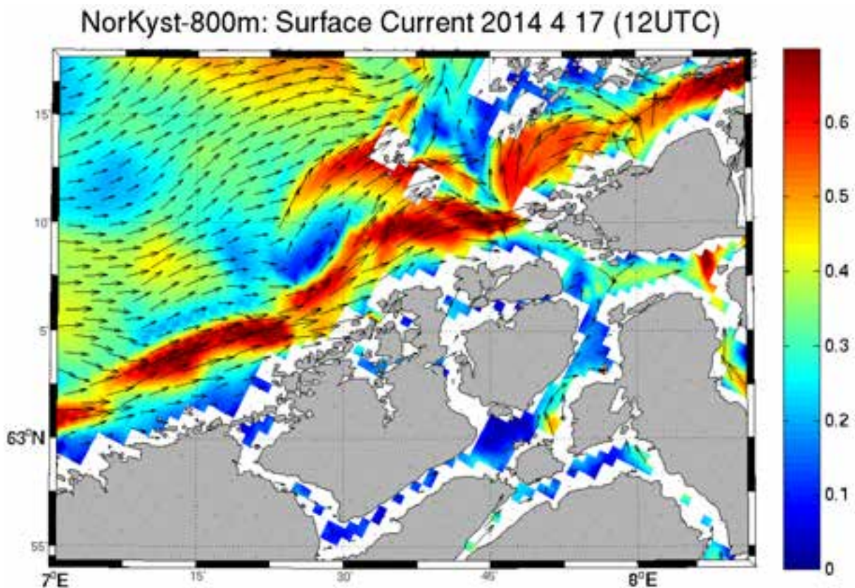
Figur 6. Strømforholdene på kysten på dagen for grunnstøtingen, simulert med Norkyst-800 modellen. Fargeskalaen angir strømhastighet (m/sek) (kilde A. Sandvik, Havforskningsinst.).
