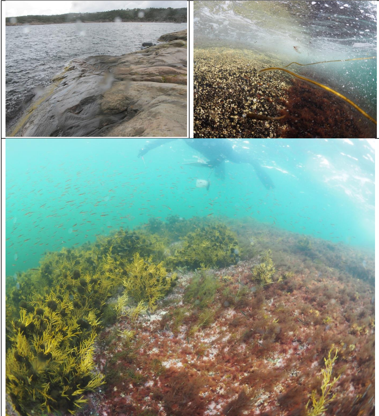
Figur 24. Stasjon 1, Ytre kyst, Risør. Bølgeeksponert stasjon dominert av skolmetang ( Halidrys siliquosa ) og små rødalger. Foto: Janne Gitmark/Maia Røst Kile.
