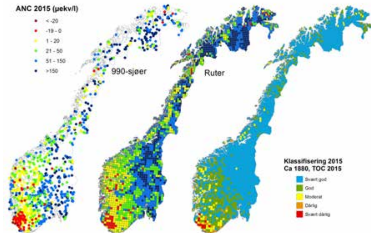
Figur 2. Modellert ANC for de 990 innsjøene (venstre), modellert ANC overført til rutene (midten) og klassifisering av forsuretilstand på rutenivå (høyre) i 2015.
