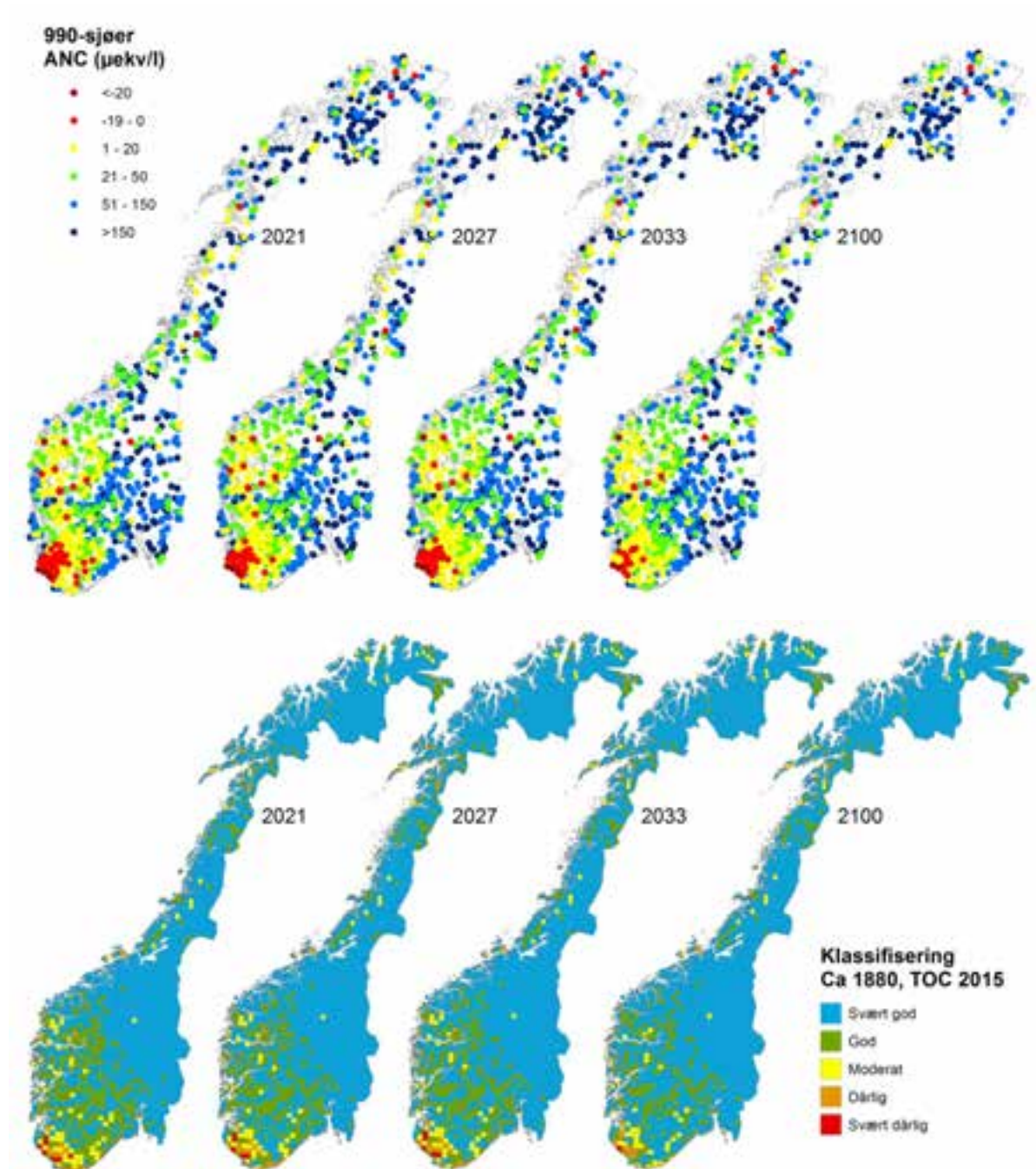
Figur 3. Modellert ANC for de 990 innsjøene (øverst) og klassifisering av forureningstilstand på rutenivå (nederst) i 2021, 2027, 2033 og 2100.
