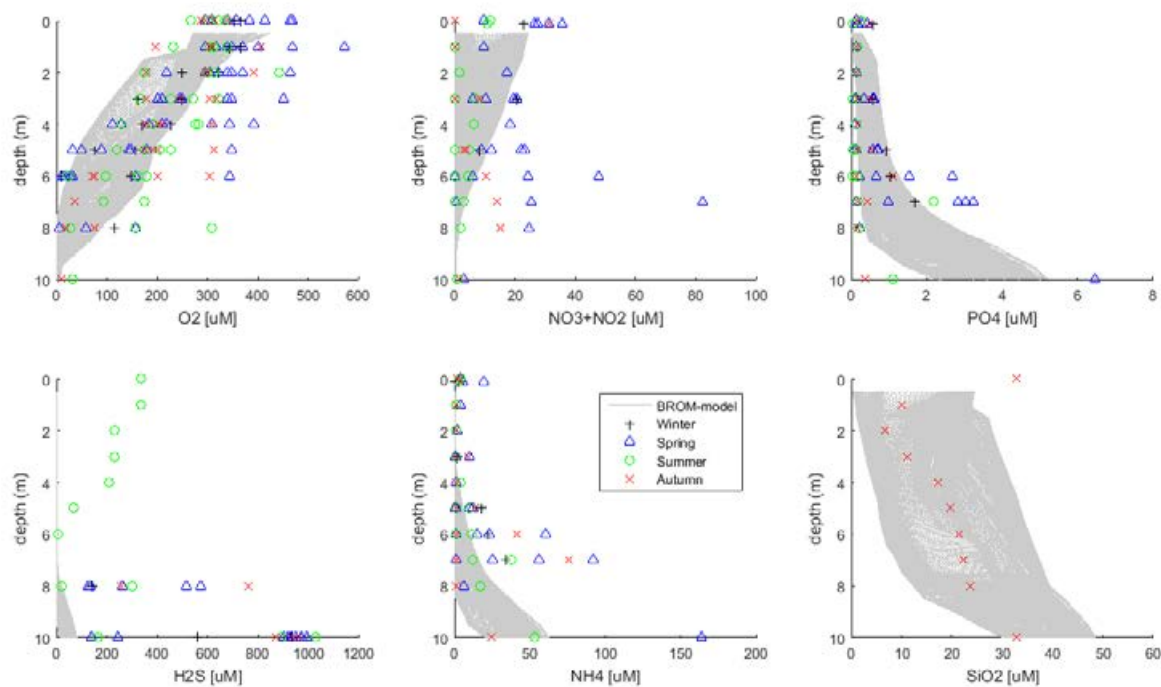
Figur 9. Modellert (grå linjer) og observert (fargede symboler) over sesongmessig variasjon i fordelingen av O 2 , NO 3 +NO 2 , PO 4 , H 2 S, NH 4 og SiO 2 i Sælenvatnet.
