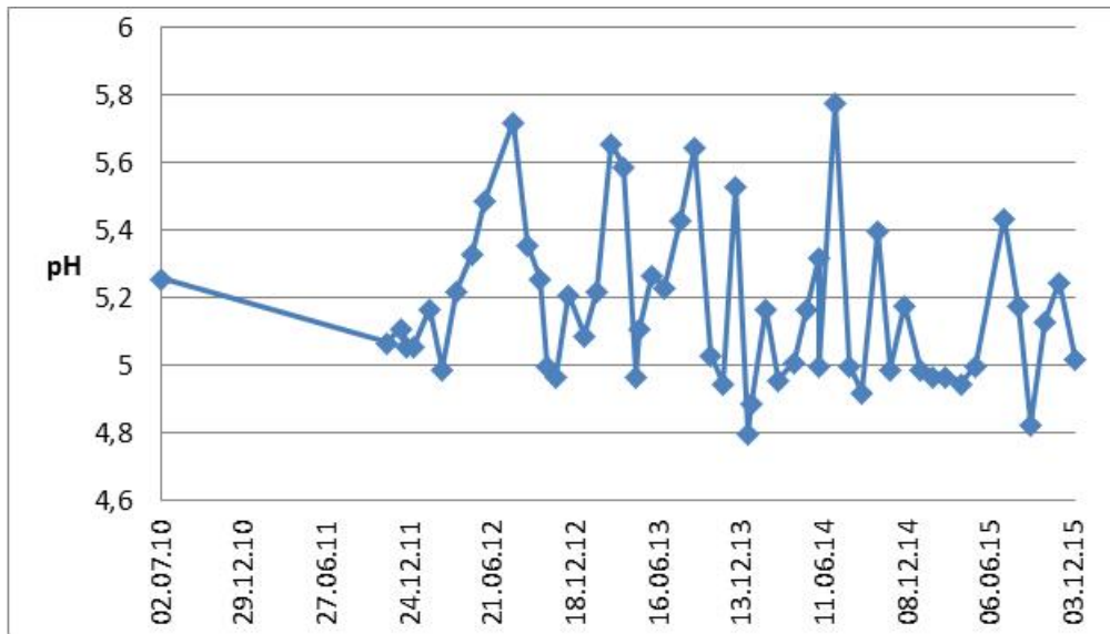
Figur 6. pH oppstrøms all kalking i Skjeggedal gjennom fem år. (Referanse: Tiltaksobservasjonen 2010-2015).
