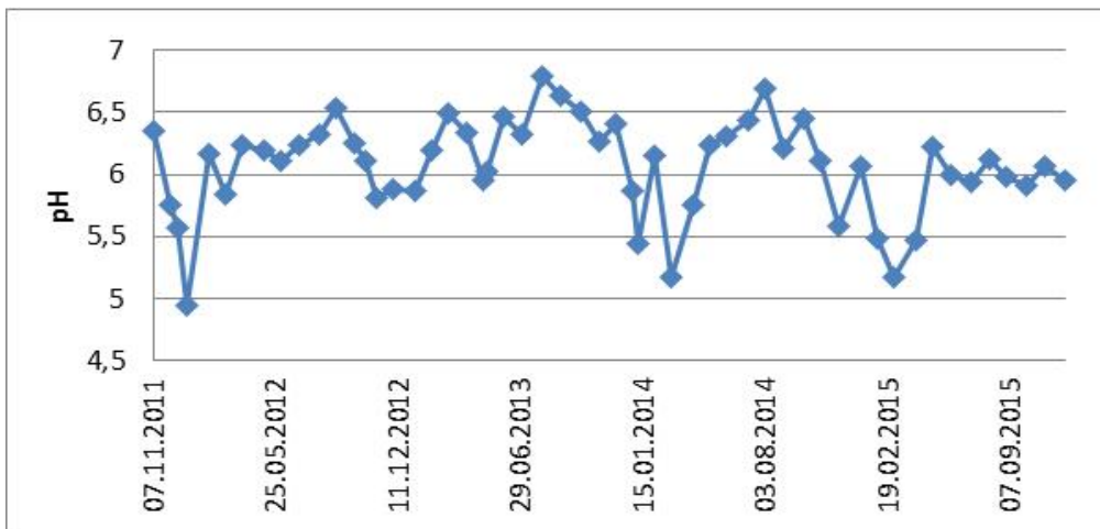
Figur 7. pH ved utløpet av Uldalsgreina ved Hanefossen gjennom fire år. Lav pH oppstår i forbindelse med flom. (Referanse: Tiltaksobservasjonen 2011-2015).
