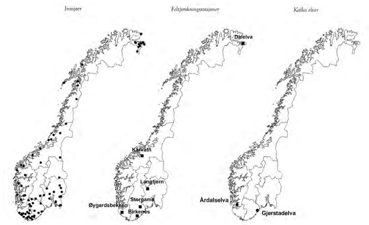
Figur 1. Lokalisering av alle de undersøkte lokalitetene i 2015 (innsjøer, elver og feltforskningsstasjoner). Linjene viser grensen til de 10 regionene (se Vedlegg A for inndeling av regioner).
