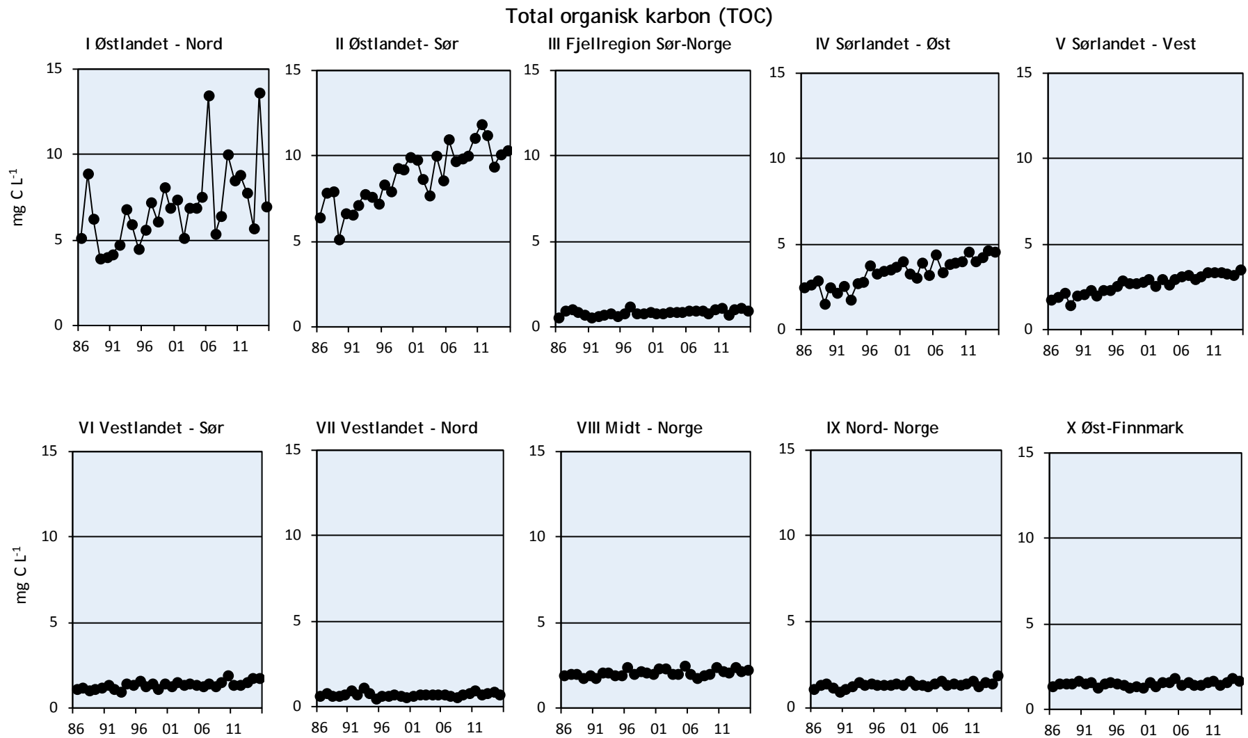
Figur 10. Trender for total organisk karbon (TOC) for innsjøer i de 10 regionene for perioden 1986-2015.
