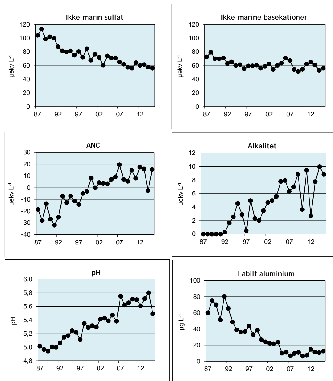
Figur 11. Forsuringsparametere for seks små vann på Jarfjordfjellet for perioden 1987-2015. Middelverdier for ikke-marin sulfat ( \text{SO}_4^* ), ikke-marine basekationer ( \text{Ca}+\text{Mg}^* ), syrenøytraliserende kapasitet (ANC), alkalitet, pH og labilt aluminium.
