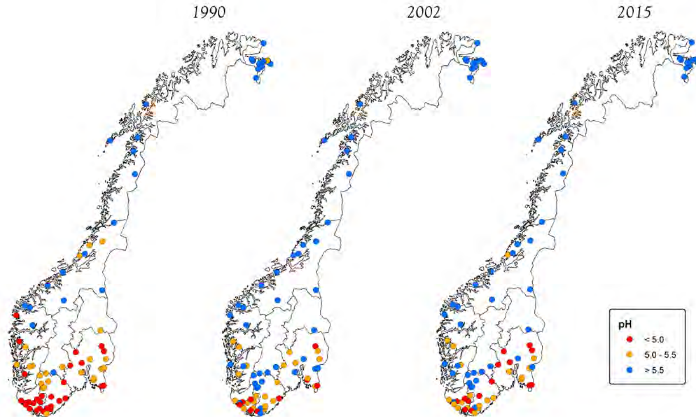
Figur 2. pH i overvåkingsinnsjøene i 1990, 2002 og 2015. Figuren illustrerer tydelig forbedringen i forurensingssituasjonen, ved at sjøene blir mindre sure (får høyere pH). Enkelte sjøer på Østlandet er fortsatt røde, og dette er forårsaket av høyt humusinnhold som gir naturlig lav pH.
