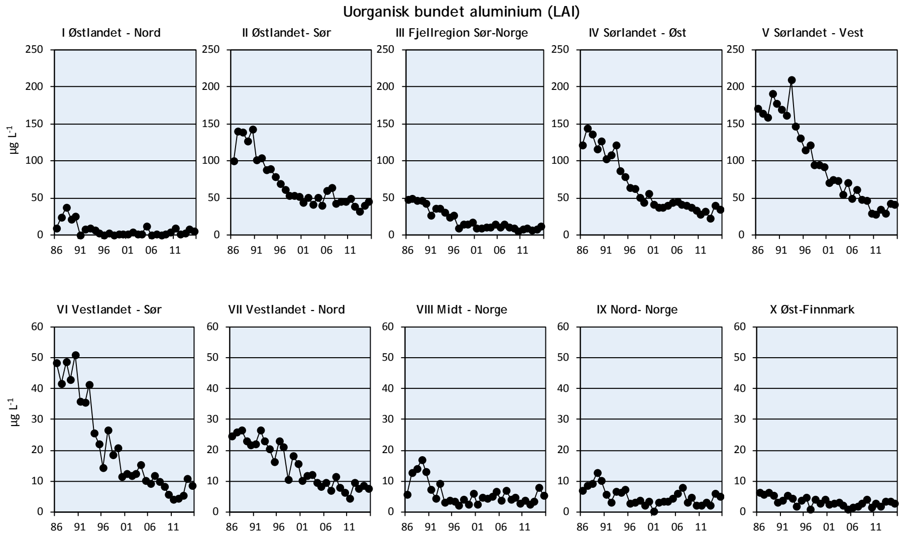
Figur 9. Trender for labilt uorganisk (bundet) aluminium (LAI) for innsjøer i de 10 regionene for perioden 1986-2015. NB! Uluk inndeling på y-aksene.
