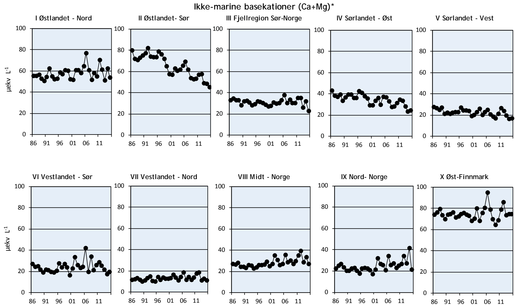
Figur 7. Trender for ikke-marine basekationer (Ca+Mg)* for innsjøer i de 10 regionene for perioden 1986-2015.
