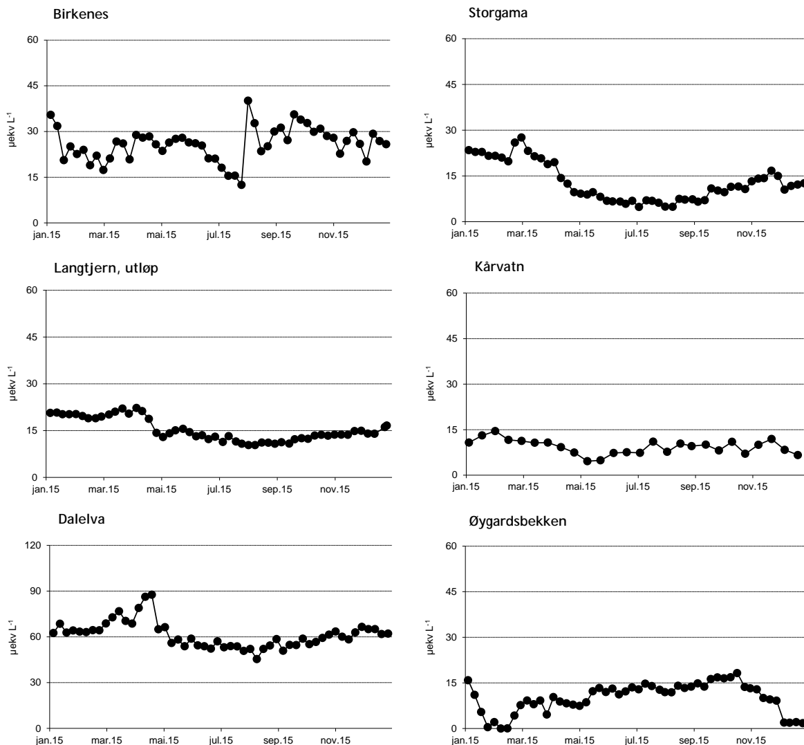
Figur 13. Sesongmessig fordeling av ikke-marin sulfat på feltforskningsstasjonene i 2015. NB! Ulik skala på y-aksene. Enhet: \mu\text{ekv L}^{-1} .
