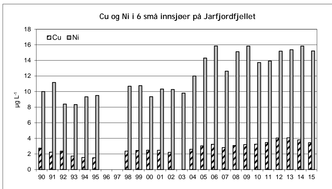
Figur 12. Årlige middelverdier for kobber og nikkel i seks små innsjøer på Jarfjordfjellet for perioden 1990-2015.
