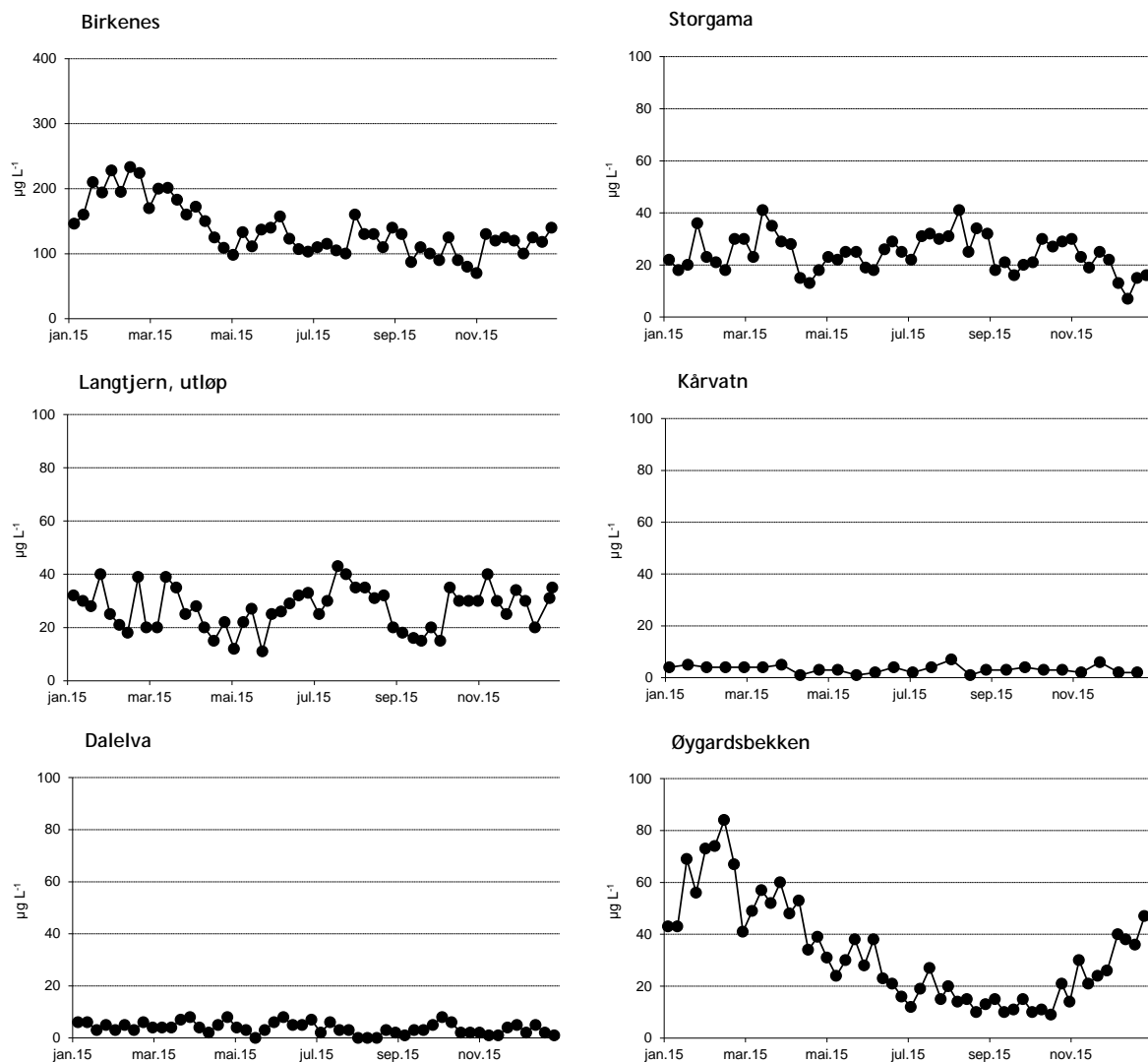
Figur 15. Sesongmessig fordeling av labilt uorganisk (bundet) aluminium (LAI) på feltforskningsstasjonene i 2015. NB! Uluk skala på y-aksene. Enhet: \mu\text{g L}^{-1} .
