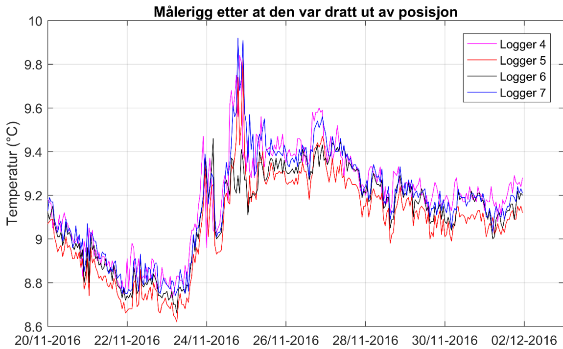
Figur 6. Temperaturmålinger fra fire av loggerne som i perioden som er vist kan antas å ha ligget på bunn og i omtrent samme dyp.
