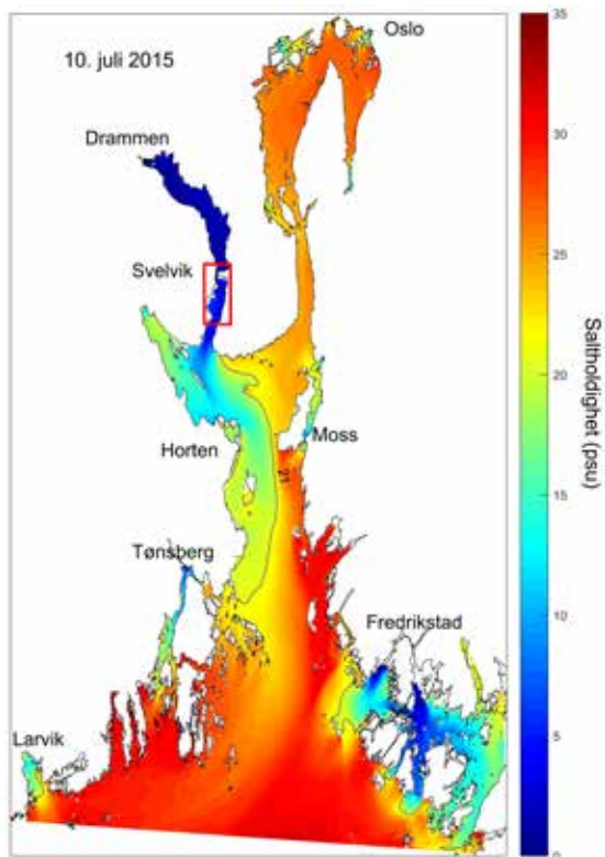
Figur 2. Eksempel på modellresultater fra FjordOs-modellen. Her vises saltholdigheten i overflatelaget i en flomsituasjon. Selv om det er et markant skille ved Drammenfjordens utløp, med betydelig saltere vann utover i fjorden, er det tydelig at Drammenselven påvirker saltholdigheten i store deler av Oslofjorden. Konturlinjen for 21 psu i saltholdighet er tegnet inn.
