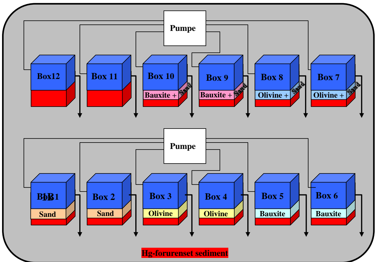
Figur 10. Illustrasjon av eksperimentelt oppsett.
