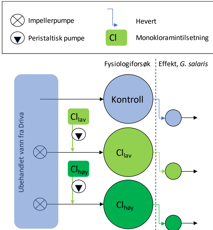
Figur 1. Skjematisk fremstilling av forsøksoppsett. Store sirkler representerer forsøkskarene der stor, voksen laks ble eksponert for klorholdig vann. Små sirkler representerer forsøkskarene der laksunger med G. salaris ble eksponert for vannet fra de store karene.
