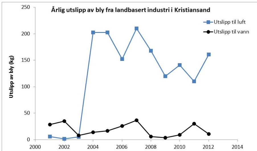
Figur 51. Årlige utslipp av Pb til luft og vann fra landbasert industri i Kristiansand i perioden 2001 til 2012. Data for figuren er hentet fra www.norskeutslipp.no .
