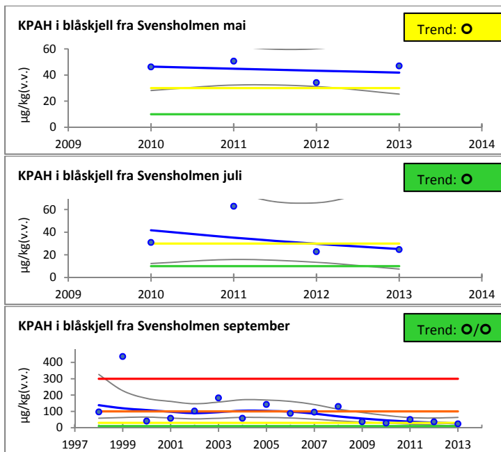
Figur 33. Nivå av KPAH ( \mu\text{g}/\text{kg v.v.} ) i blåskjell fra Svensholmen i mai, juli og september. Horisontale fargede linjer markerer grenseverdi for Miljødirektoratets tilstandsklasse (Tabell 5). Merk ulike skala på y-aksen.
