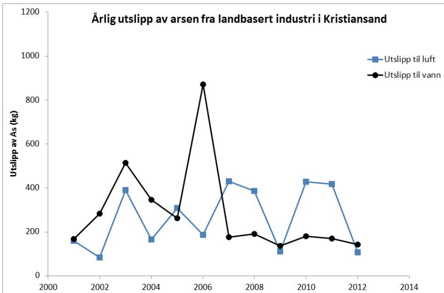
Figur 52. Årlige utslipp av As til luft og vann fra landbasert industri i Kristiansand i perioden 2001 til 2012. Data for figuren er hentet fra www.norskeutslipp.no .
