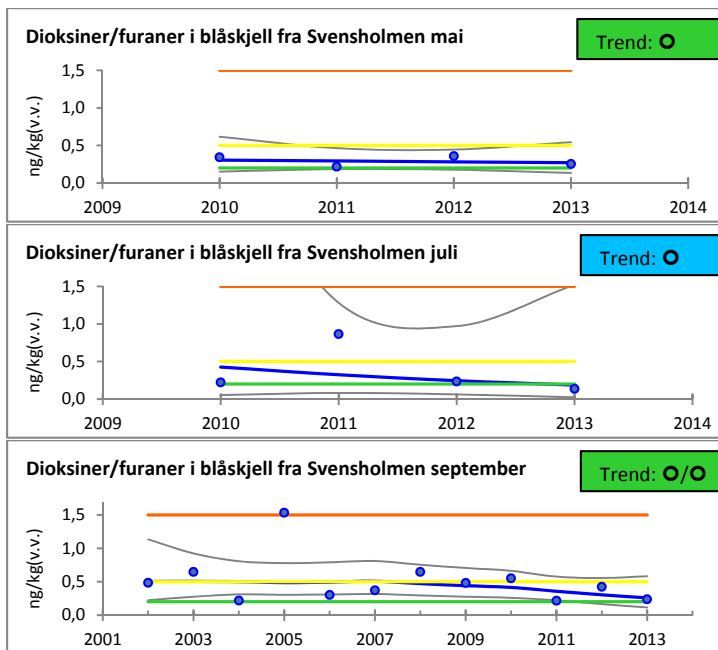
Figur 44. Toksitetsekvivalenter for dioksiner/furaner (TE PCDD/F ng/kg v.v.) i blåskjell fra Svensholmen i mai, juli og september. Horisontale fargede linjer markerer grenseverdi for Miljødirektoratets tilstandsklasse (Tabell 5).
