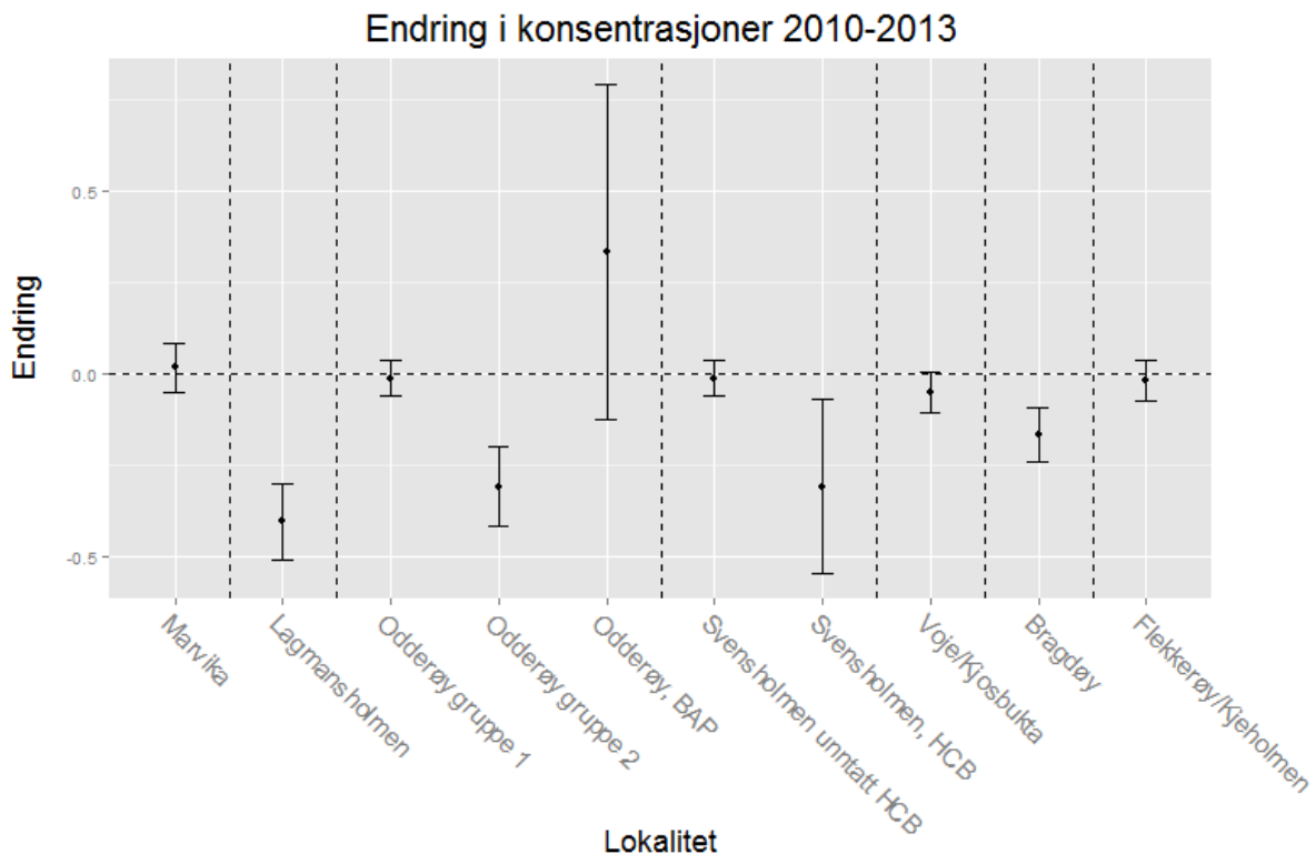
Figur 57. Tidstrender på hver stasjon i fireårsperioden 2010-2013. Punktene viser estimert trend, mens de lodrette linjene viser ca. 95 % usikkerhet ( 2 \cdot SE ). Positive verdier viser en økning av konsentrasjoner, negative verdier viser en nedgang. Odderøy gruppe 1 inkluderer de fleste metallene og noen organiske miljøgifter (Al, As, Cd, Co, Cu, Fe, Hg, Ni, Pb, Si, Zn, TBT, PAH, KPAH, PCB-7, non-ortho PCB, TE dioksiner). Odderøy gruppe 2 inkluderer Cr, Ag, Ca, HCB, HCB, TE dioksiner/furaner, TE furaner. Alle HCB-verdiene var under deteksjonsgrensen.
