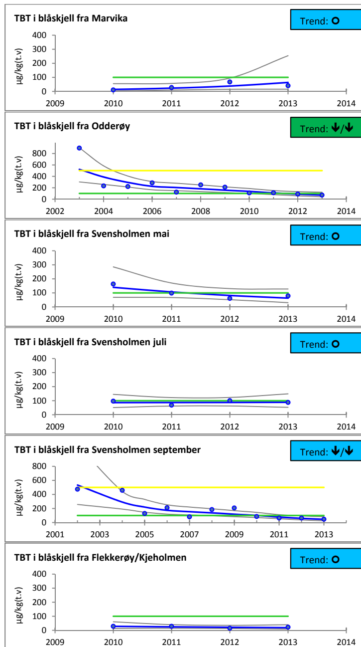
Figur 36. TBT-innhold ( \mu\text{g}/\text{kg t.v.} ) i blåskjell innsamlet på høsten i tillegg til mai og juli ved Svensholmen. Horisontale fargede linjer markerer grenseverdi for Miljødirektoratets tilstandsklasse (Tabell 5). Resultatene er basert på én blandprøve per stasjon bortsett fra ved Odderøy og Svensholmen til og med 2011, hvor det ble analysert to blandprøver for TBT. Merk ulik skala på y-aksen.
