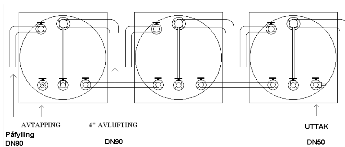
Figur 1. Prinsippskisse av anlegg som er koblet sammen i serie med tre enheter. Innbyrdes avstand mellom containerne bør være minimum 1 meter.
