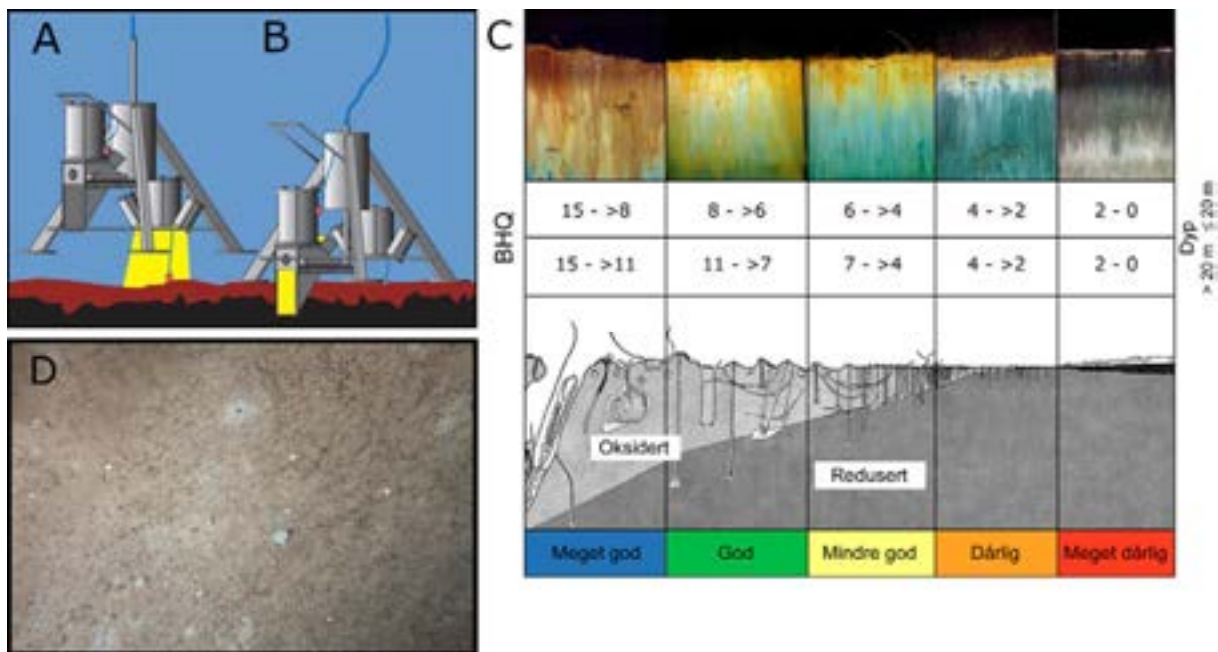
Figur 4. Prinsippskisse for SPI-kamera og bildeanalyse. (A) Rigg over bunnen. Gult antyder at det tas bilde av overflaten. (B) Kamera med prismet som har trengt ned i sedimentet og SPI bildet eksponeres. (C) Figuren viser en modell av endringer i faunatype fra upåvirkede bunnsedimenter med en rik, dyptgravende fauna (Meget god) til en grunnlevende, fattig fauna i påvirkede områder (Meget dårlig). Sedimentprofilbildet er vist i toppen av figuren, der brunt farget sediment indikerer oksidert, bioturbert sediment mens sortfarget sediment indikerer reduserte forhold. Grenseverdier for BHQ-miljøkvalitetsindeks for vanddyb \leq 20 meter og > 20 m i samme skala som benyttes for marine sedimenter i EUs vanddirektiv (Pearson og Rosenberg, 1978, Nilsson og Rosenberg, 1997, Rosenberg et al., 2004, Nilsson og Rosenberg, 2006). (D) Eksempel av et overflatebilde med strukturer og børstemarkrør synlig. Figur hentet fra NIVAs faktaark om SPI.
