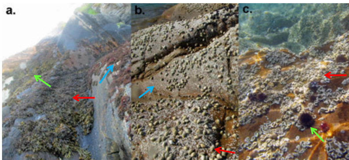
Figur 12. Glomfjorden. a. Stasjon 2. Saуетang (blå pil), spiraltang (rød pil) og en blanding av blæretang og grisetang (grønn pil) på fjell. b. Stasjon 3. Purpursnegl (rød pil) og rur (blå pil) på fjell. c. Stasjon 3. Drøbakkråkeboller (grønn pil) og trekantmark (rød pil) på fjell.
