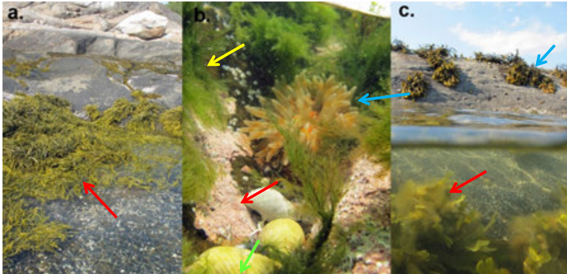
Figur 13. Nordfoldfjorden. a. Stasjon 1. Grisetang (rød pil) på fjell. b. Stasjon 2. Vanlig grønndusk ( Cladophora rupestris ) (gul pil), fjæresjørøse (blå pil) og purpursnegl (grønn pil) på fjell med endel skorpeformete røde kalkalger ( Coralliniacea indet.) (rød pil) c. Stasjon 3. Spiraltang (blå pil) og sagtang ( Fucus serratus ) med perlesli ( Pylaiella littoralis ) på fjell.
