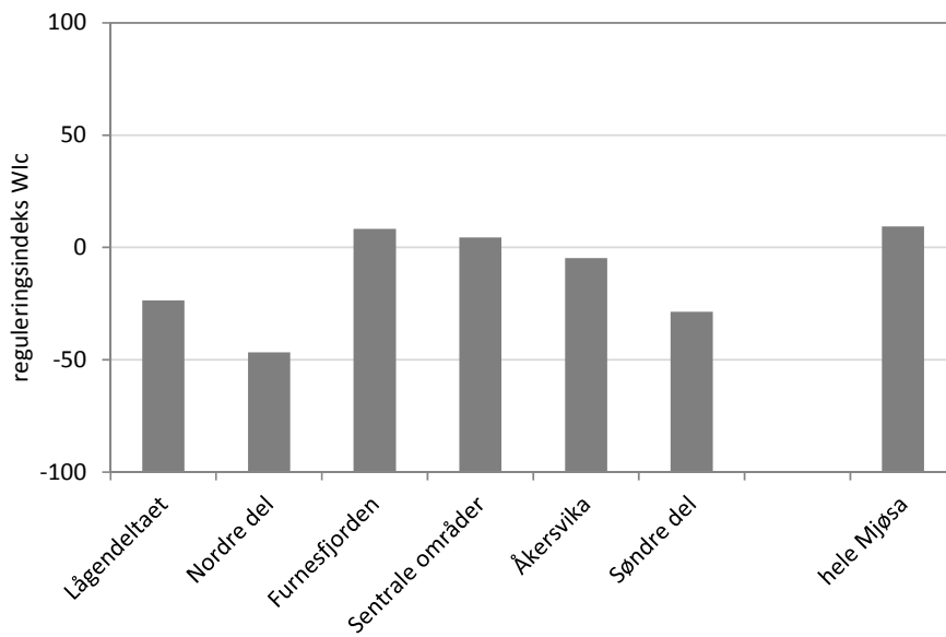
Figur 6. Økologisk tilstand for vannvegetasjonen (basert på WIC-indeksen, foreløpig) i ulike områder av Mjøsa (se tabell 1). Klassegrensene iht. Direktoratgruppen vanndirektivet (2013).
