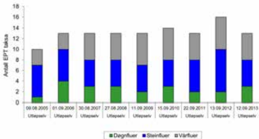
Figur 8. Antall EPT taksa (art/slekt/familie) i utløpselv fra Flensjøen fra 2005 til 2012. Sparkeprøver 3×1 min.
