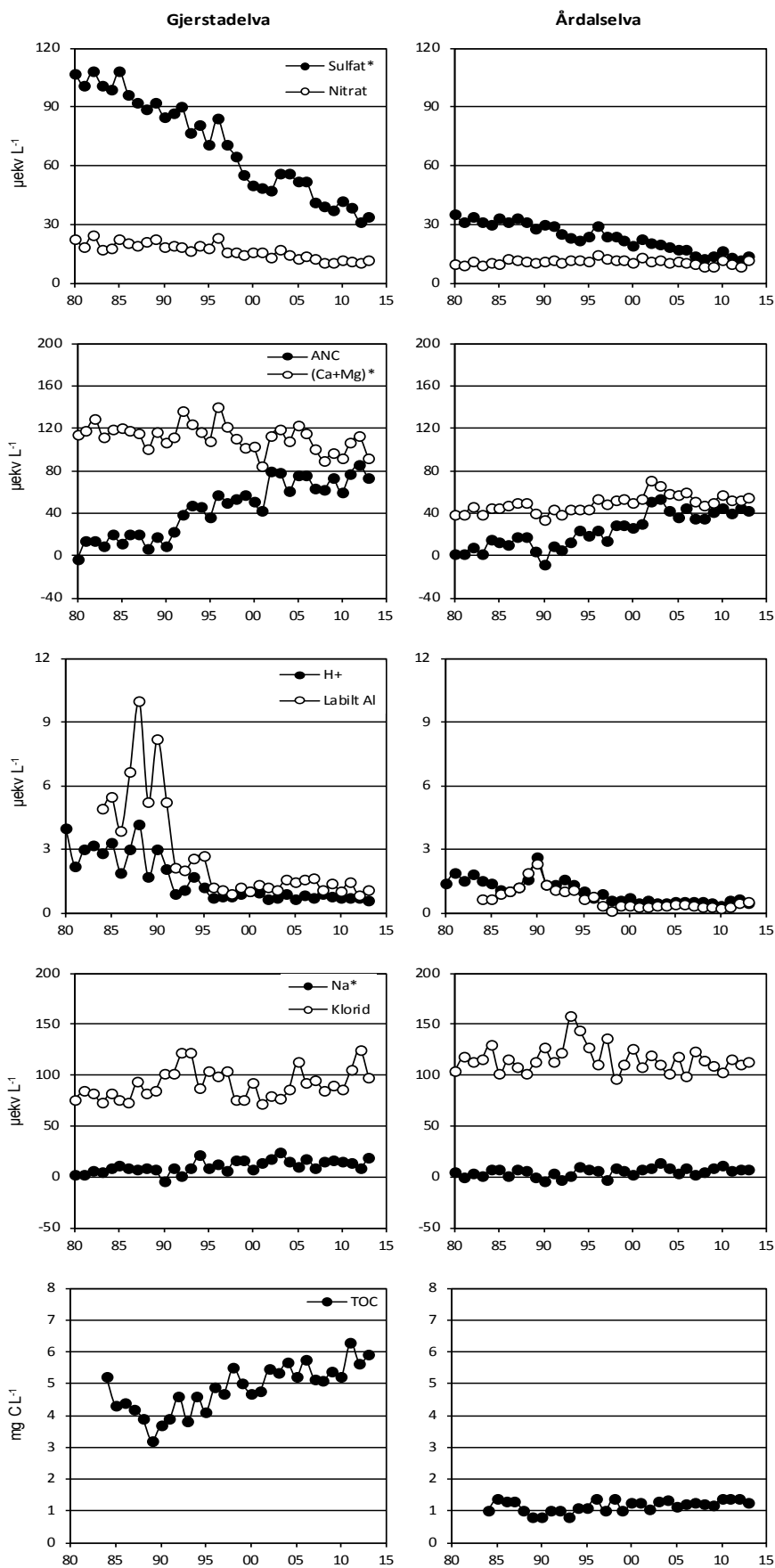
Figur 25. Årsmiddelverdier av utvalgte parametere i Gjerstadelva og Årdalselva for perioden 1980-2013.
