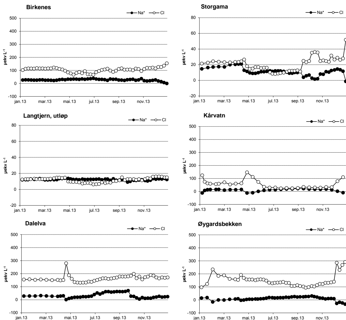
Figur 16. Sesongmessig fordeling av klorid og ikke-marin natrium på feltforskningsstasjonene i 2013. Ikke-marin natrium ● og klorid ○. NB! Ulik skala på y-aksene. Enhhet: µekv L -1 .
