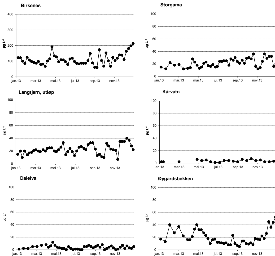
Figur 15. Sesongmessig fordeling av labilt uorganisk (bundet) aluminium (LAI) på feltforskningsstasjonene i 2013. NB! Uluk skala på y-aksene. Enhet: \mu\text{g L}^{-1} .
