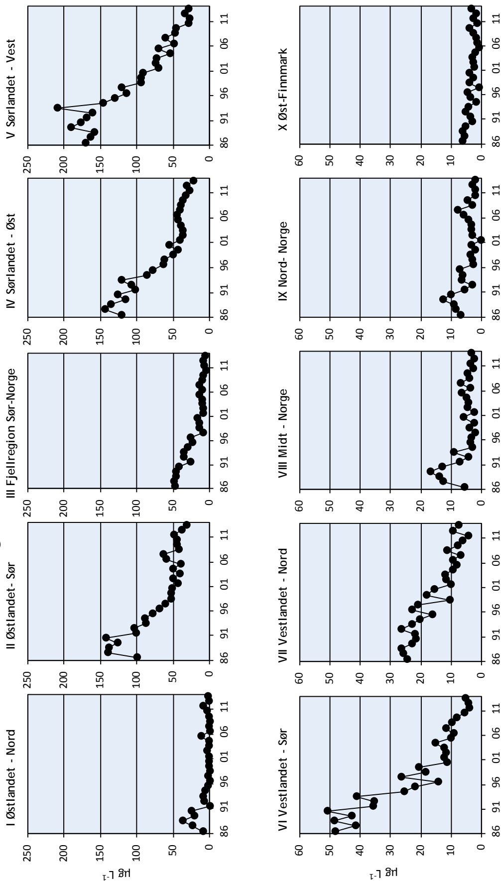
Figur 9. Trender i labilt uorganisk (bundet) aluminium (LAI) for perioden 1986-2013 for innsjøer i de 10 regionene. NBI Ulik inndeling på y-aksene.
