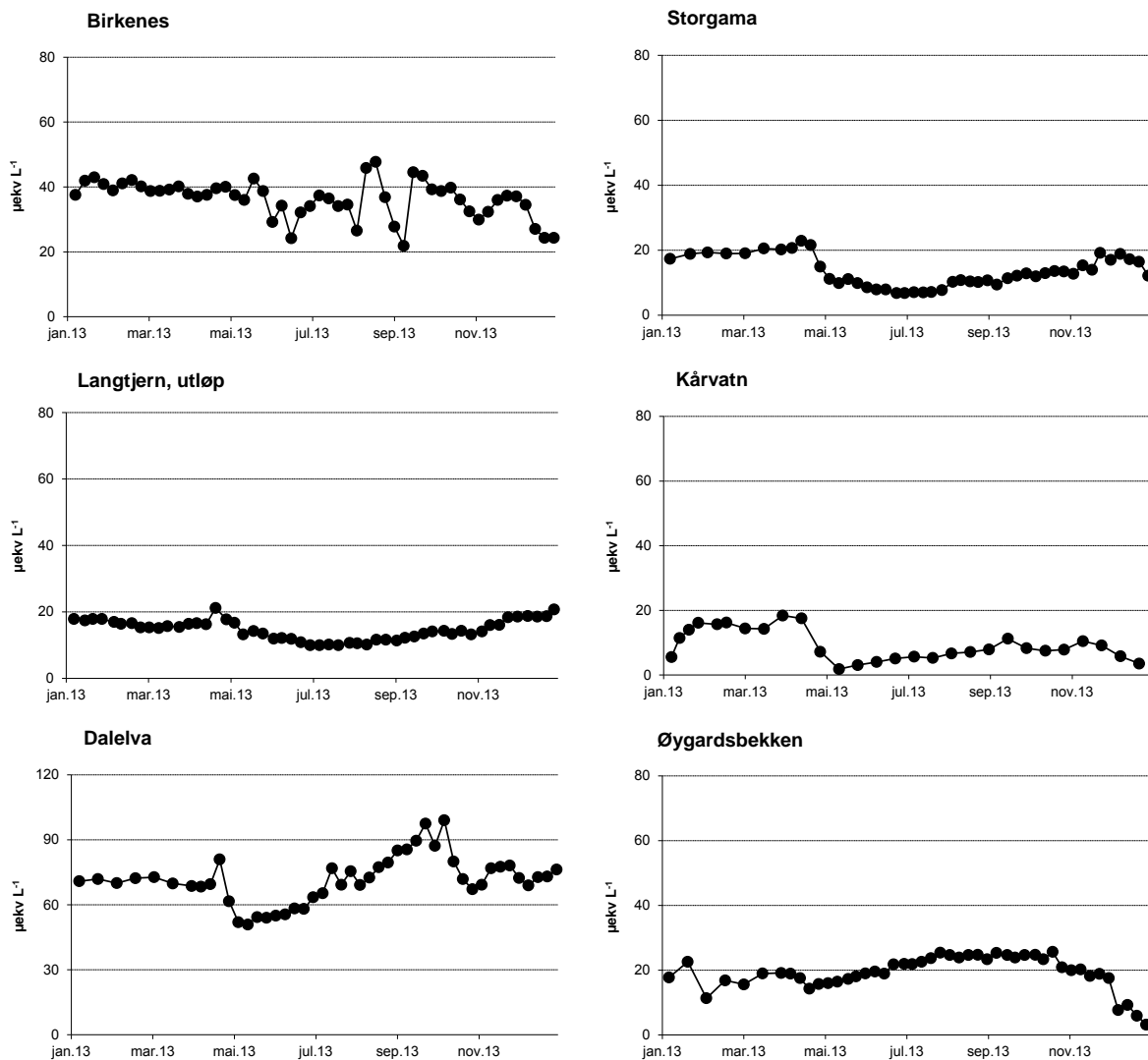
Figur 13. Sesongmessig fordeling av ikke-marin sulfat på feltforskningsstasjonene i 2013. Enhet: \mu\text{ekv L}^{-1} .
