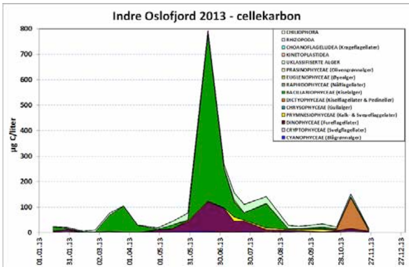
Figur 17. Algebiomasse i form av cellekarbon ( \mu\text{g C/L} ) for 2013. Prøver fra ca. 4 meters dyp i Vestfjorden automatisk samlet inn med MS «Color Festival» ved Steilene.
