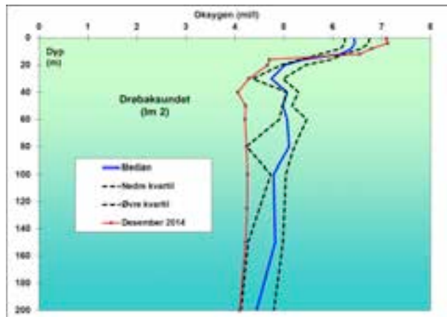
Figur 12. Konsentrasjonen av oksygen i desember 2014 i Drøbaksundet i ulike dyp. I figuren er også medianverdier for årene 1973-1982 (inkludert nedre og øvre kvartil) inntegnet.
