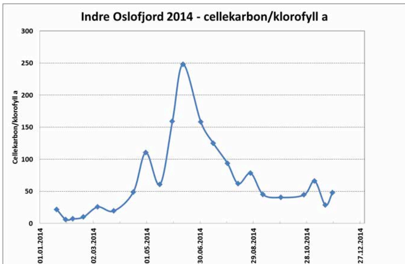
Figur 18. Utviklingen av forholdet mellom cellekarbon og klorofyll a gjennom året på stasjon Dk1 i 2014.
