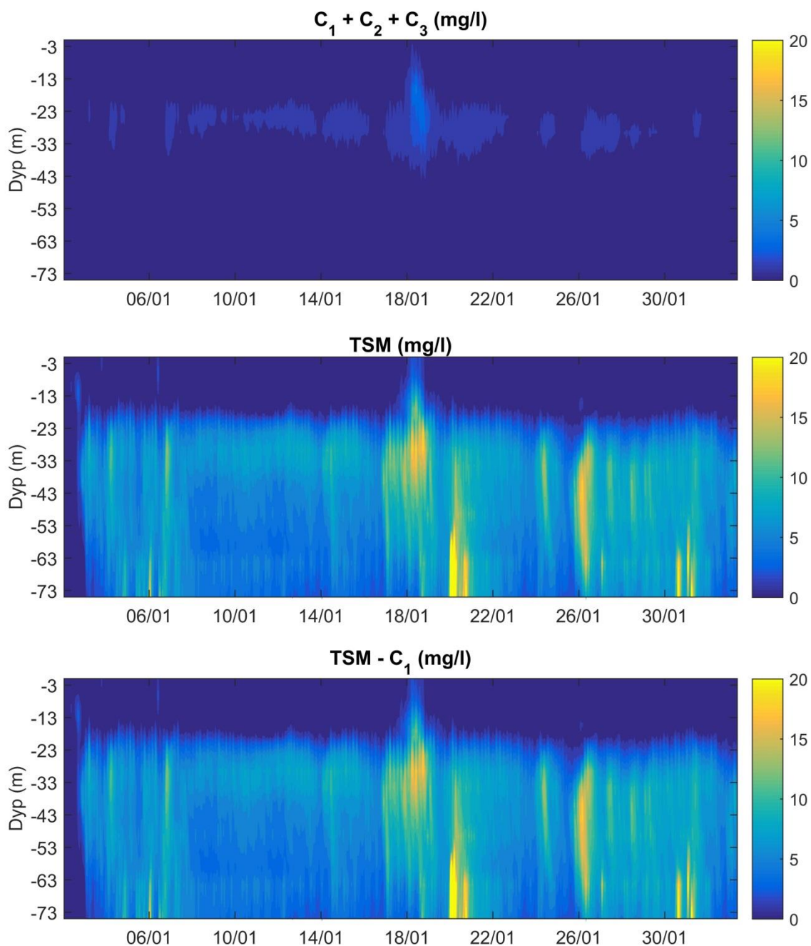
Figur 15. Partikkelkonsentrasjon på stasjon 2. Øverst vises summen av de tre minste partikkelklassene med kornstørrelse mindre enn 16 \mu\text{m} . I midten vises summen av alle de ni partikkelklassene. Nederst vises effekten av å fjerne partikler mindre enn 4 \mu\text{m} . Kornfordeling med mindre finstoff er brukt (jmfør Figur 9 ).
