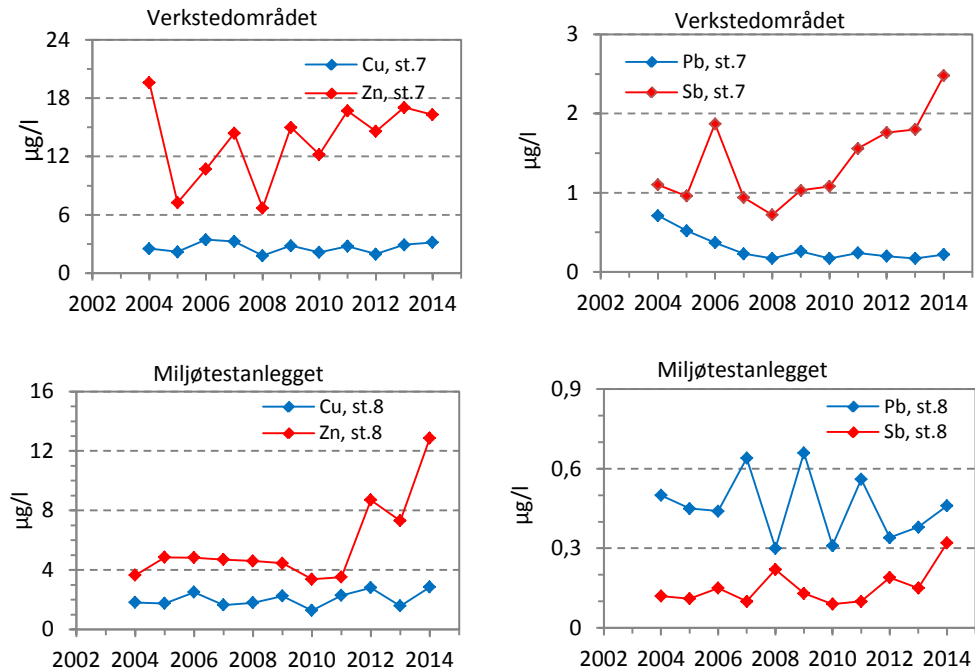
Figur 7. Middelkonsentrasjoner av kobber (Cu), bly (Pb), sink (Zn) og antimon (Sb) i bekken fra verkstedområdet og fra miljøtestanlegget
