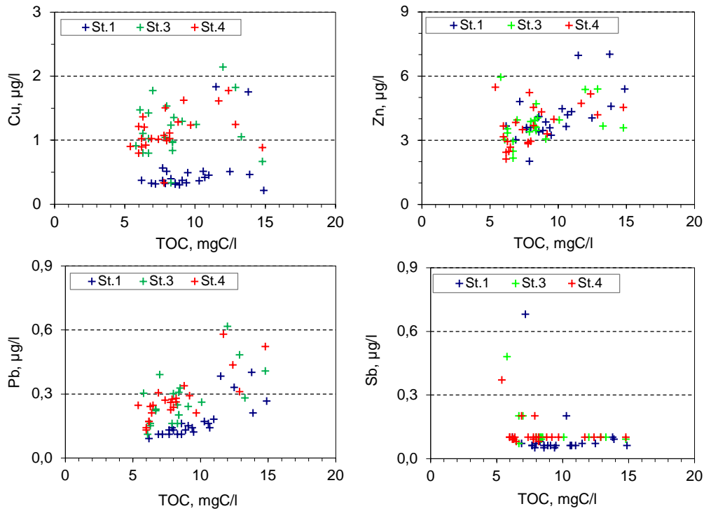
Figur 5. Sammenhengen mellom TOC (totalt organisk karbon) og konsentrasjoner av metaller på ulike stasjoner i Veltmannåa (2007-2012).
