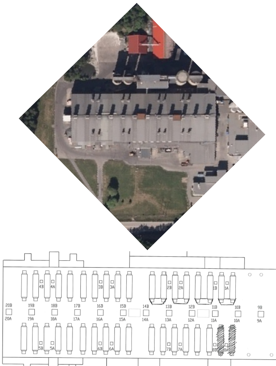
Figur 2. Ovnshuset med piper (kvadrater i skissen med nr 9-20 er sentralt plassert og to rekker med nr. 1-8 er plassert på sidene) og ovner (sylinderformede). Den sentralt plasserte renna i betong (ikke inntegnet) går under gulvnivået under sentralpipene.
