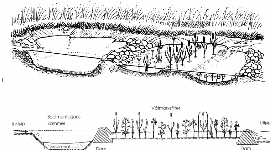
Figur 11. Prinsippskisser av en fangdam
