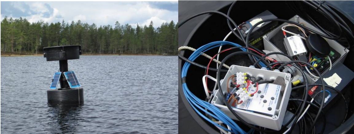
Figur 1. Bøye med sensorer i flere dyp, elektronikk for automatisk oversendelse av data samt strømforstyrning fra solceller.
