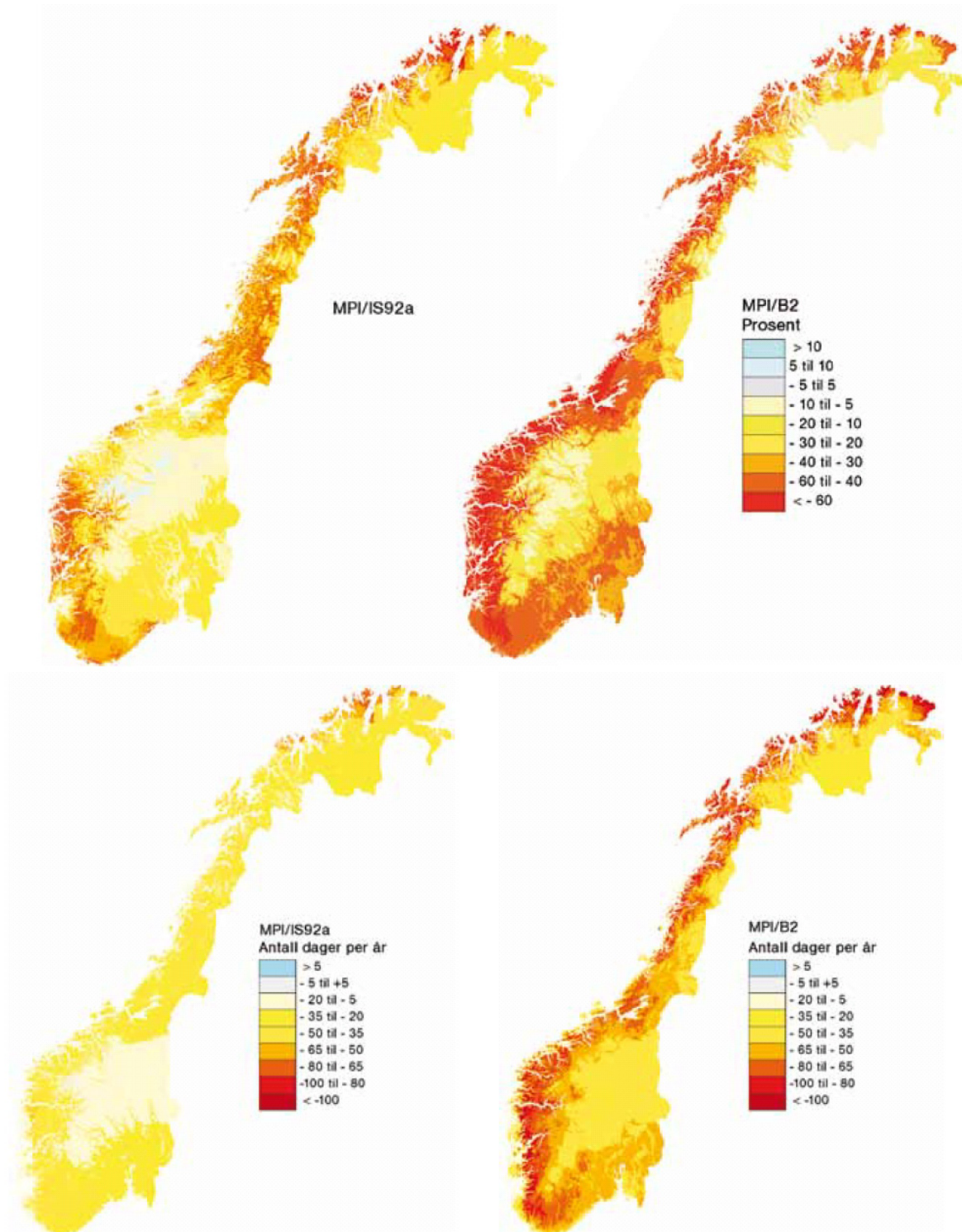
Figur 9. Prosentvis endring i maksimalt snømagasin i kort 2030-49 (øverst til venstre) og lang framskrivningsperiode 2071-2100 (øverst til høyre) relativt til perioden 1961-1990 og endring i antall dager med snødekke i kort (nederst til venstre) og lang framskrivningsperiode nederst til høyre i forhold til perioden 1961-1990.
