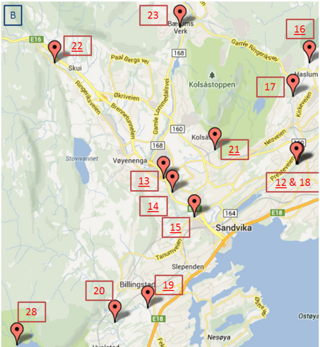
Figur 9. Kart over delområde B, med prøvepunktets nummer i følge tabell 1. Understrekede nummer ble prøvetatt både vår og høst, ellers bare vår.
