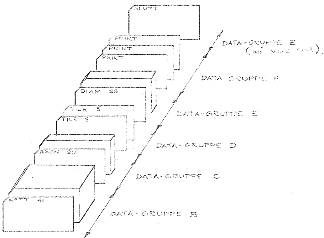
Fig. 7 Datagruppeeksempler
