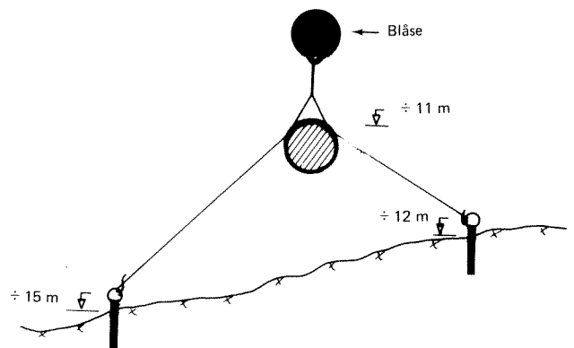
Fig. 64. Utløpsledning montert svevende over bunnen.
