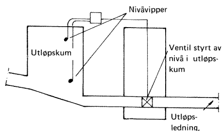
Fig. 85. Hydraulisk styring av ventil på utløpsledningen sikrer spyling.
