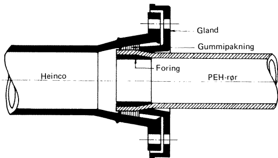
Fig. 37. Ferdig montert Heinco-PEH skjøte.
