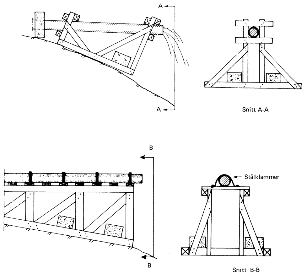
Fig. 79. Ende av utløpsledning montert på belastet treramme.
