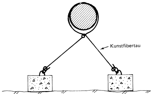
Fig. 66. Sveveledning forankret med tau til lodd på bunnen.
