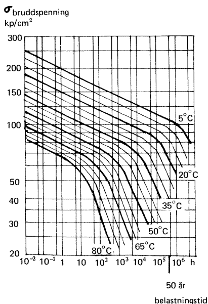
Fig. 36. Spennings-tidskurver for PEH-rør, Hostalen GM 5010.
