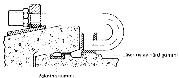
Fig. 49. O-ringtettning med strekkklave for betongrør.
