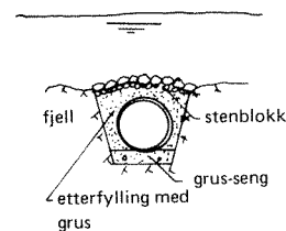
Fig. 69. Utløpsledning lagt i grøft og overdekket.
