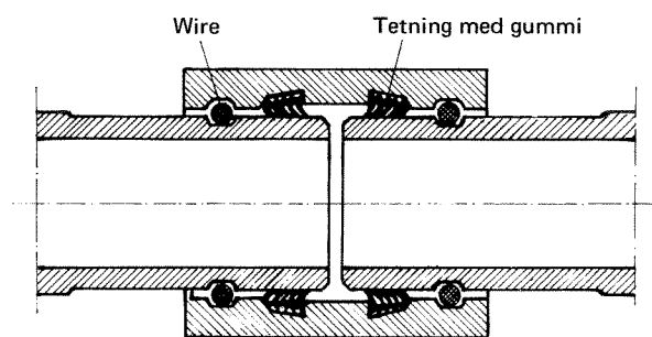
Fig. 46. Asbestsementrør med strekkfast skjøt ZOK.
