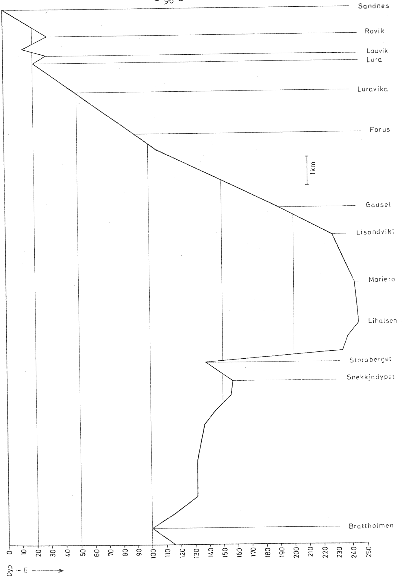
Fig.4 Bunnprofil av Gandstjard fra Sandnes til Høgsfjord/Horgefjord
