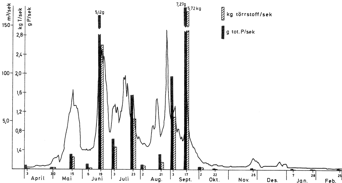
Fig.26 Bövra 1974/1975
