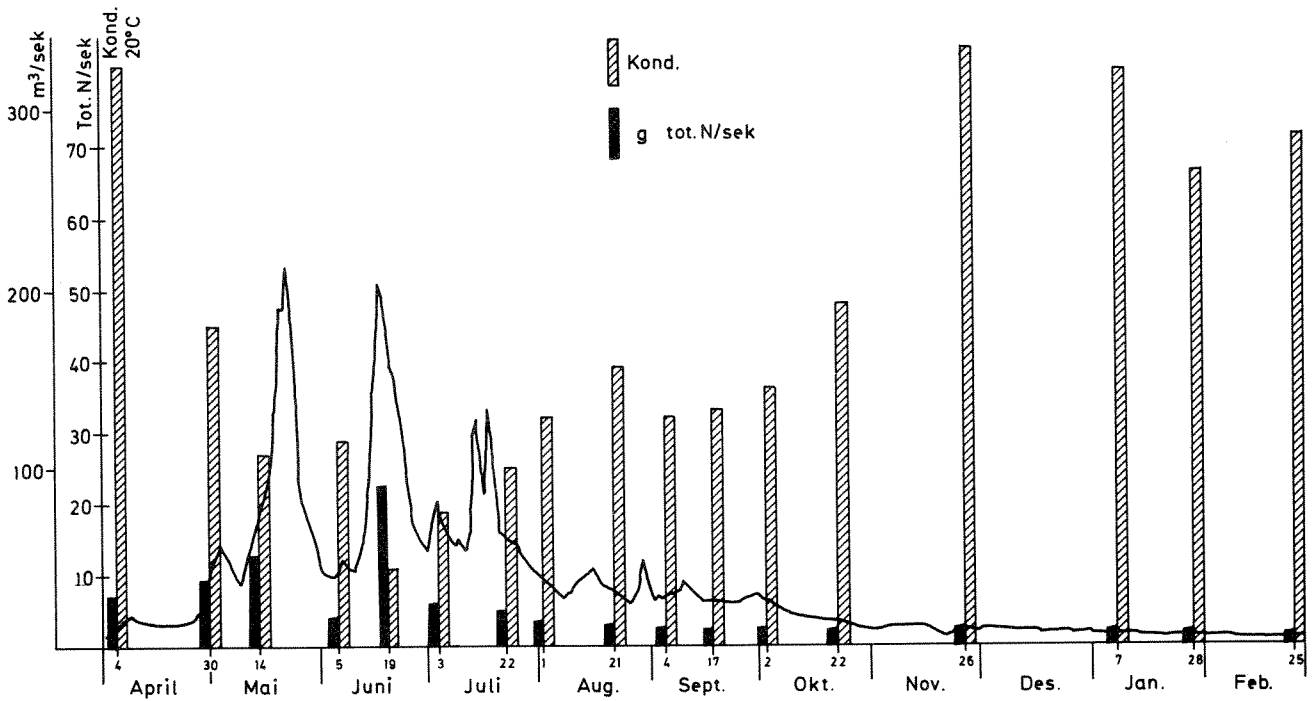
Fig.29 Lågen v/Sel 1974/1975
