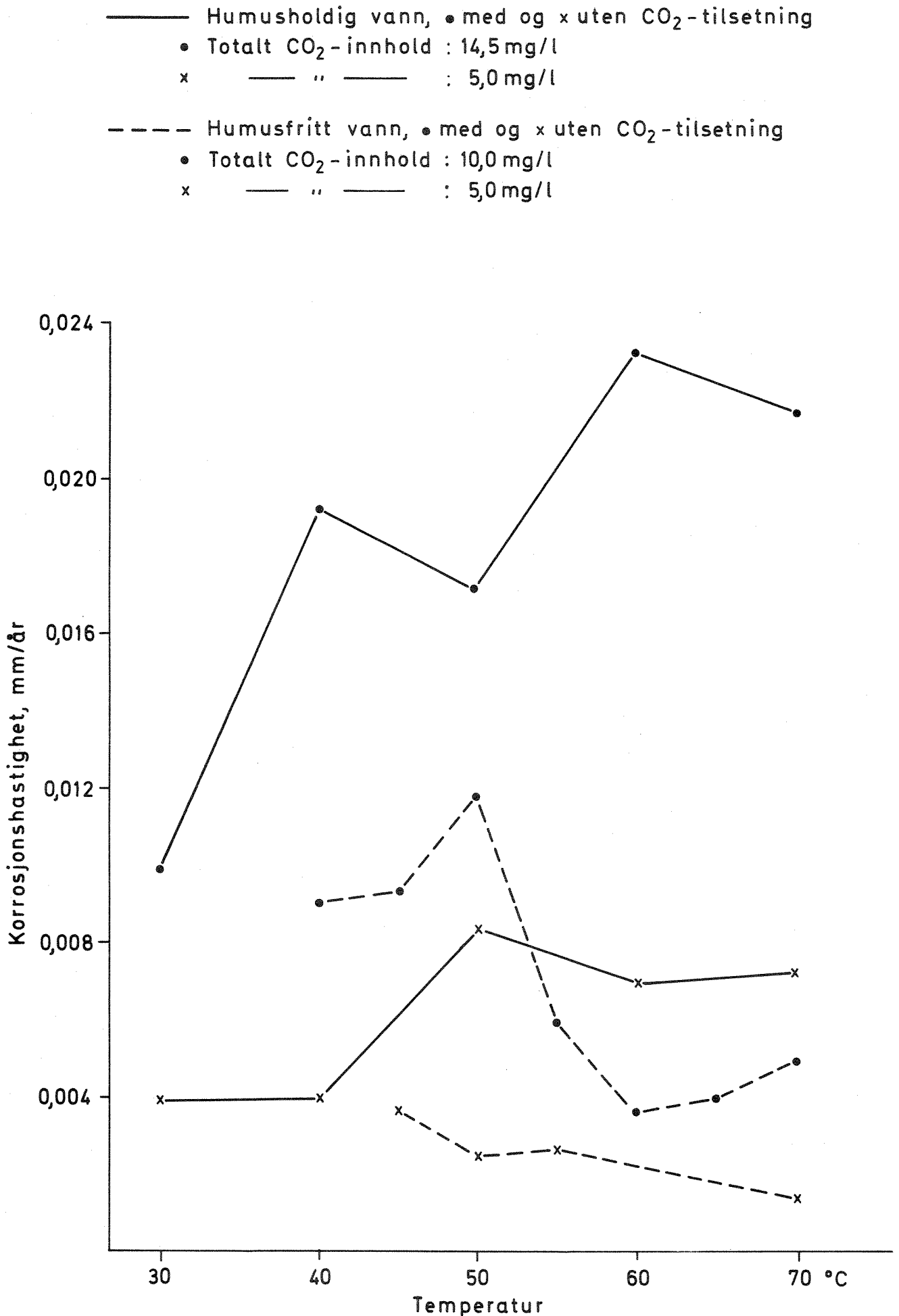
Fig.1 Korrosjon på kobber som funksjon av temperatur
