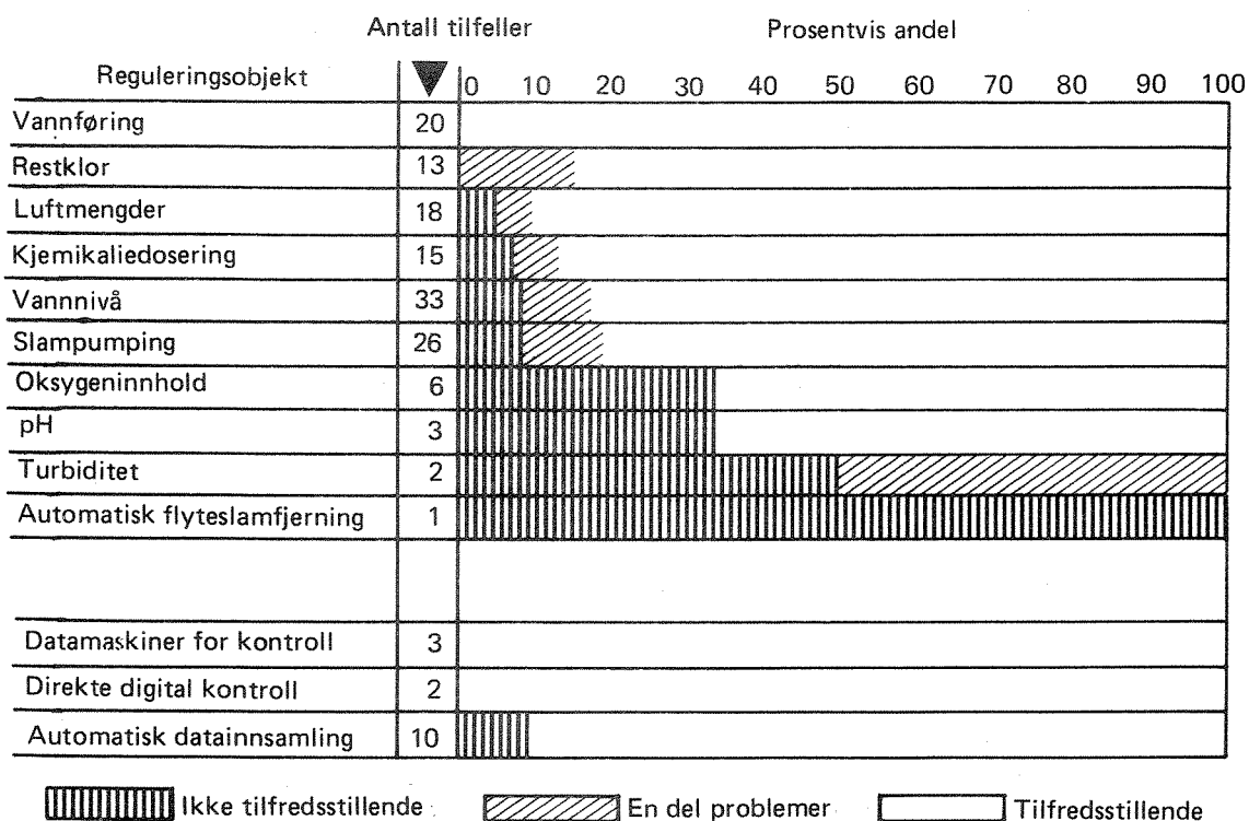
Figur 11. Sammenheng av driftserfaringer med ulike individuelle reguleringssløyfer ved 50 amerikanske renseanlegg (2).
