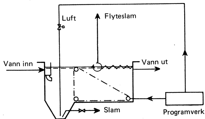
Figur 5. Forsedimenteringsbasseng med kjedeskrape.
