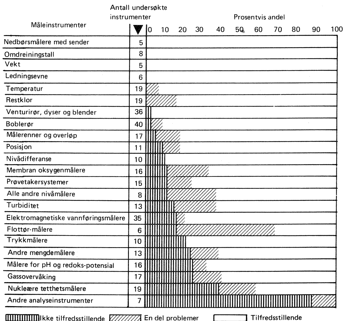
Figur 10. Driftserfaringer med ulike måleinstrumenter ved 50 amerikanske renseanlegg (2).
