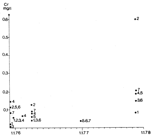
Fig. 14. Konsentrasjon av krom i sigevannet.
