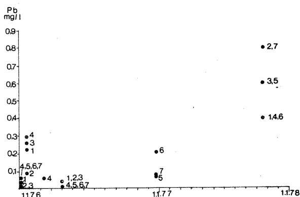
Fig. 16. Konsentrasjon av bly i sigevannet.
