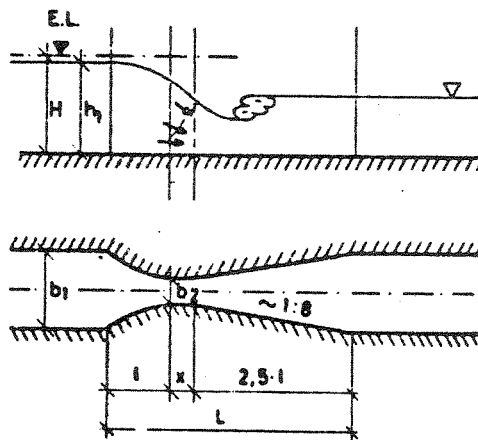
Fig. 10 Venturikanal. (3).
