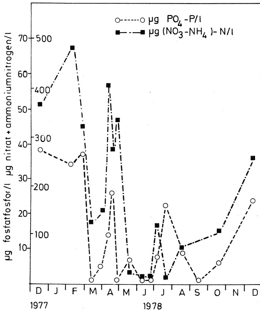
Fig. 21. Variasjon i klorofyll-a og siktedyp (øverst) og nitrat + ammonium og fosfat (nederst) på St. EP-1 (BUNNEFJORDEN) i 1978.
