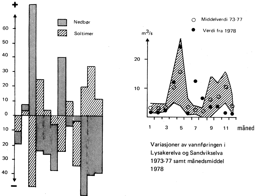
Soltimer og nedbør (mm) på Blindern, Oslo i 1978 som avvik fra perioden 1956-70 resp. perioden 1931-60 (Data fra meteorologisk institutt).
