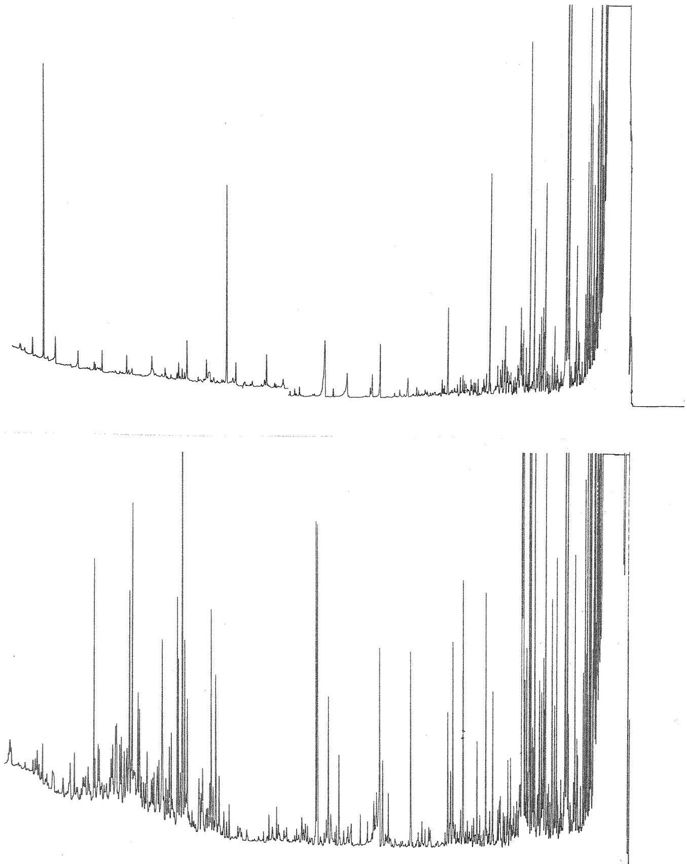
Fig. 4. Glasskapillær-gasskromatografi av upolare forbindelser ved st. 7 og 8.
