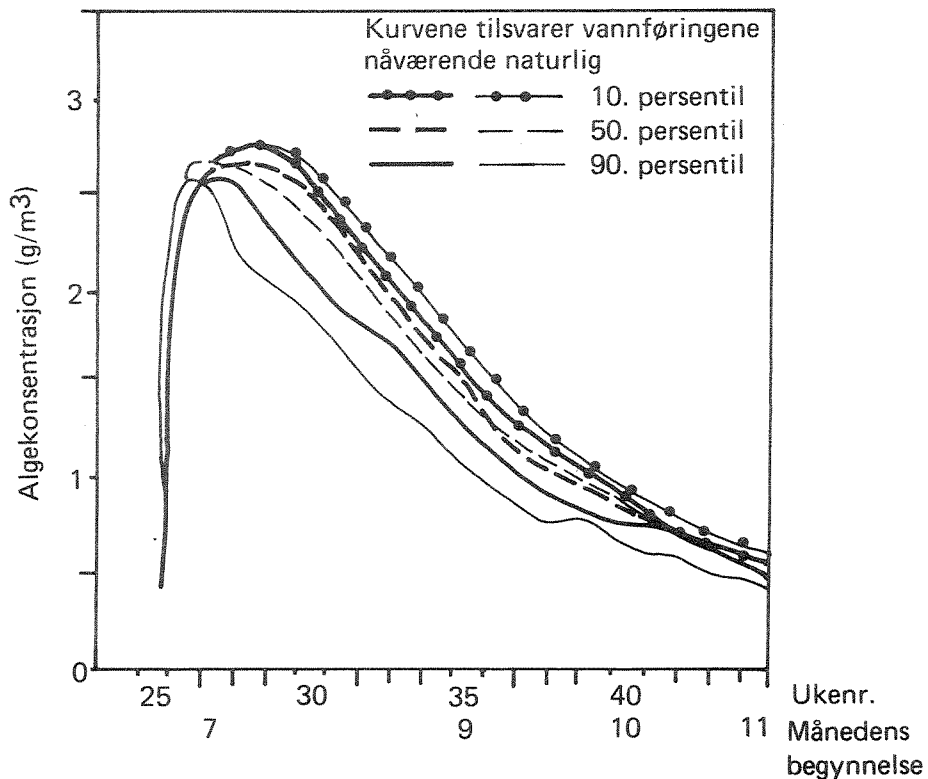
Fig. Al.1-7. Algevekst ved nåværende (tykk strek) og naturlig (tynn strek) vannføring og belastning på 230 tonn fosfor pr. år.
