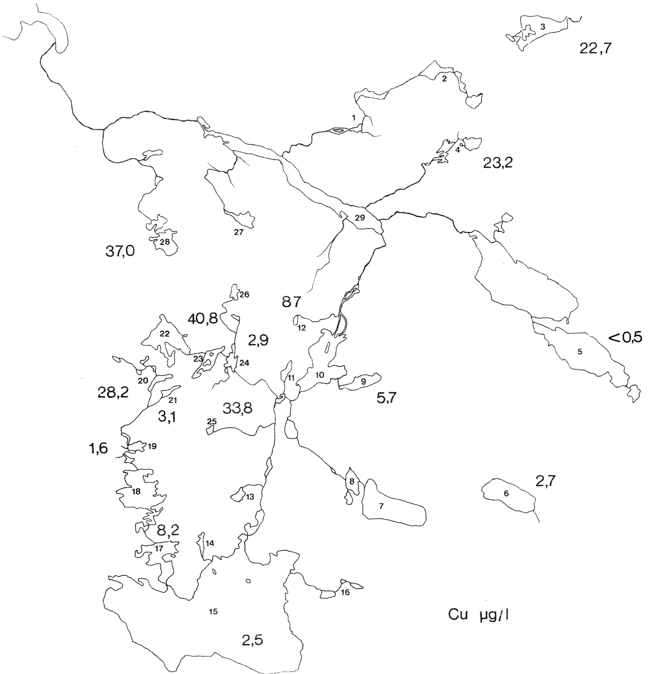
Fig. 9. Innsjøenes kobberkonsentrasjon.
