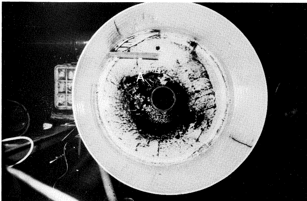
Fig. 3. Hvirveloverløp uten overløpsarrangement, sett ovenfra (forsøksenhet med diameter 1,15 m).
