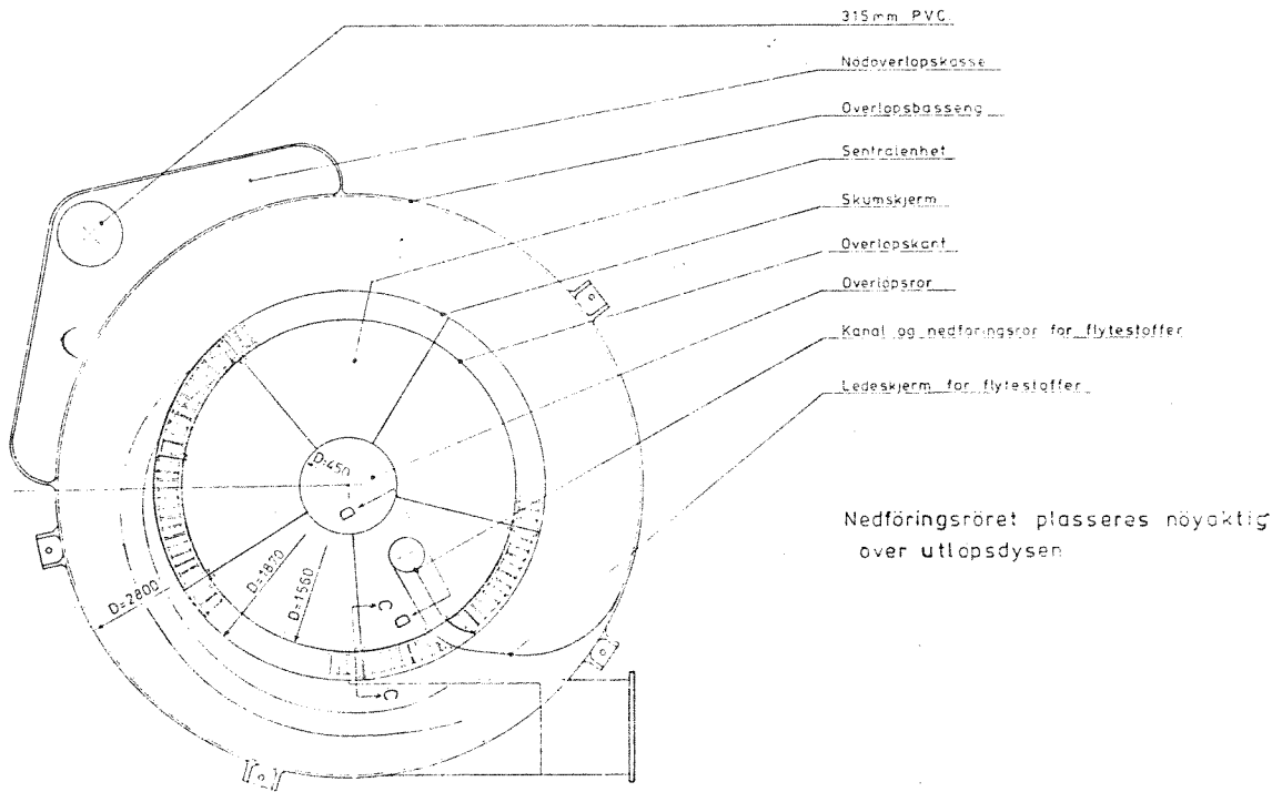
Fig. 17. Overflowbasseng med sentral overflowenhet.
