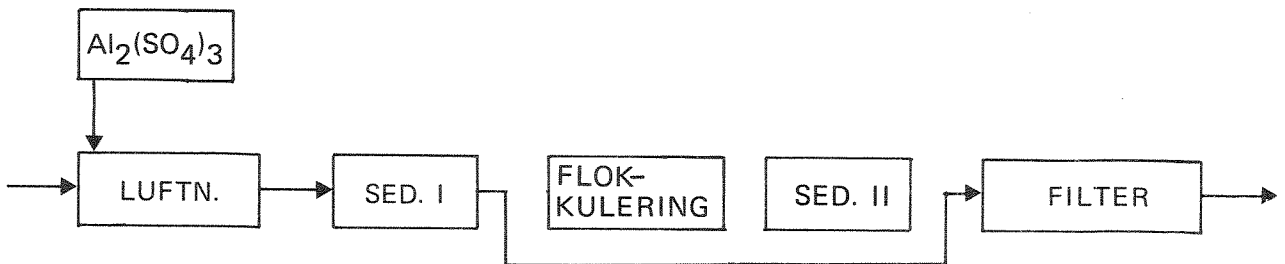
Fig. B/9 Simultanfelling med aluminiumsulfat og sluttfiltrering
