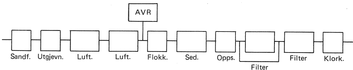
Fig. C/4. HOVEMOEN KLOAKKRENSSEANLEGG Simultanfelling med aluminiumsulfat (AVR).
