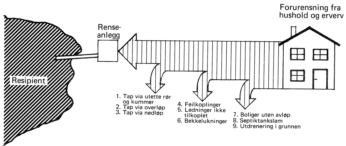
Figur 10. Ulike former for "lekkasjer" i et avløpsnett
