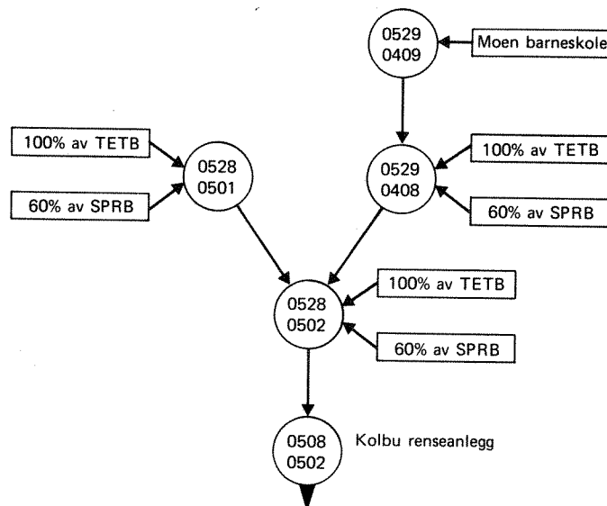
Figur 51. Kolbu rensanlegg
